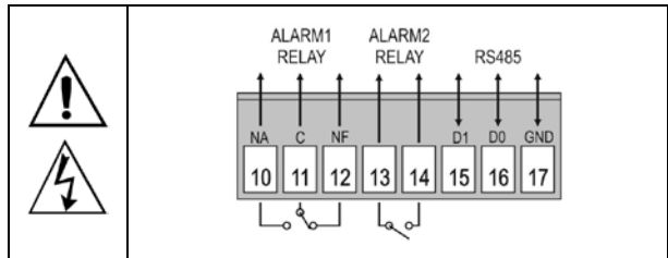
Figura 02 - Conexões de alarmes e comunicação serial
