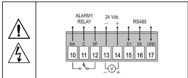
Figura 04 - Conexões de alarme, fonte auxiliar e comunicação
