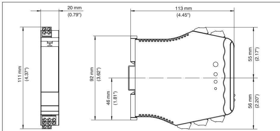
Fig. 54: Dimensões VEGATOR 122
