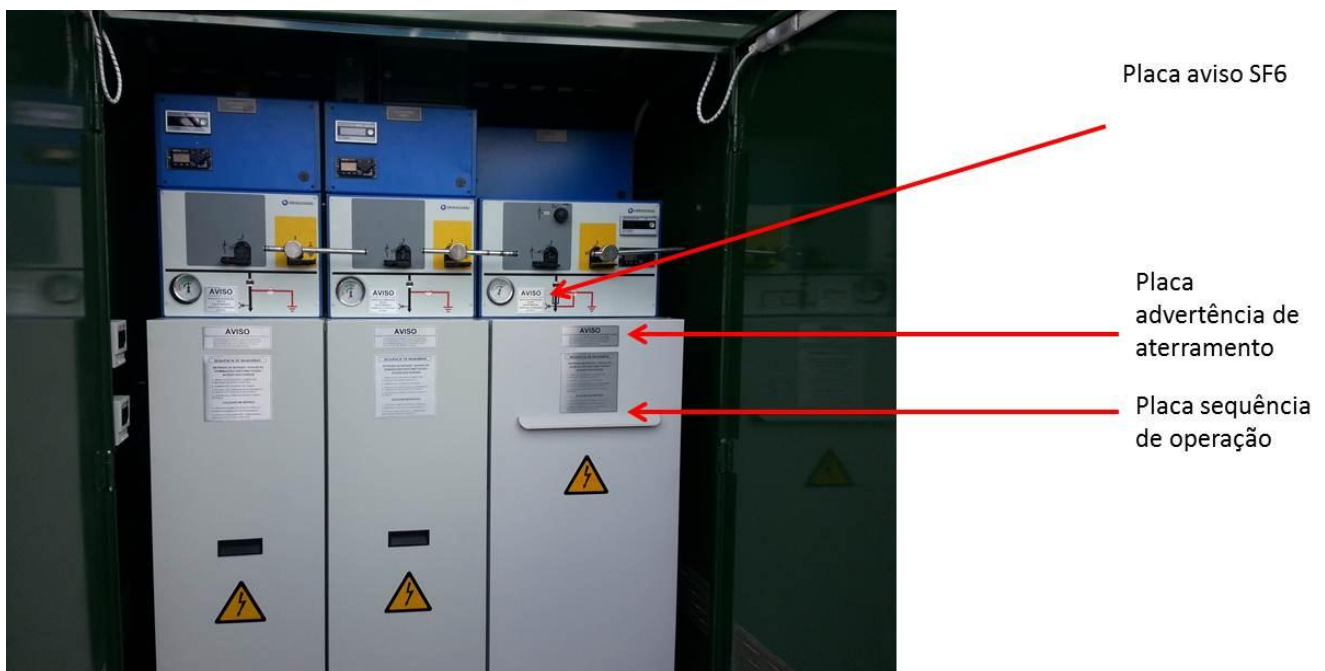
Figura 1 - Exemplo de Localização das Placas de Advertência e Operação
