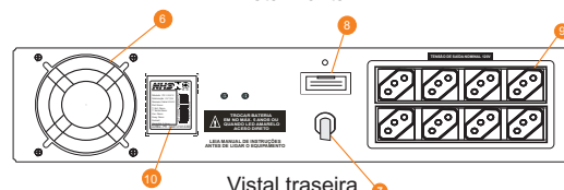
Vista traseira
