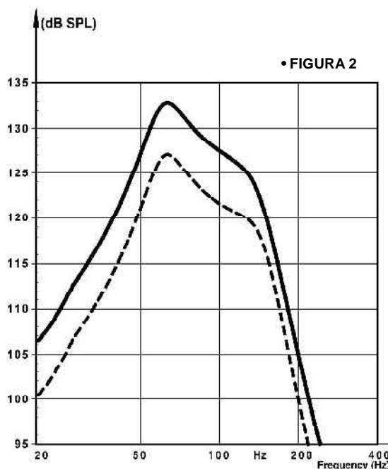
Curvas de resposta de frequência da caixa acústica S-BASS P-18 , quando conectada no sistema ativo de subwoofer S-BASS 1000 A / S-BASS 1000 A - 2G , ou recebendo amplificação externa alternativa específica de subwoofer, nas condições estabelecidas nos “Pré-requisitos Técnicos”, páginas 3 e 4.
