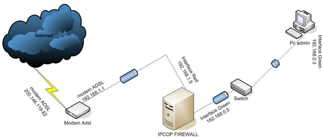
Figura 2 Diagrama detalhado da rede
