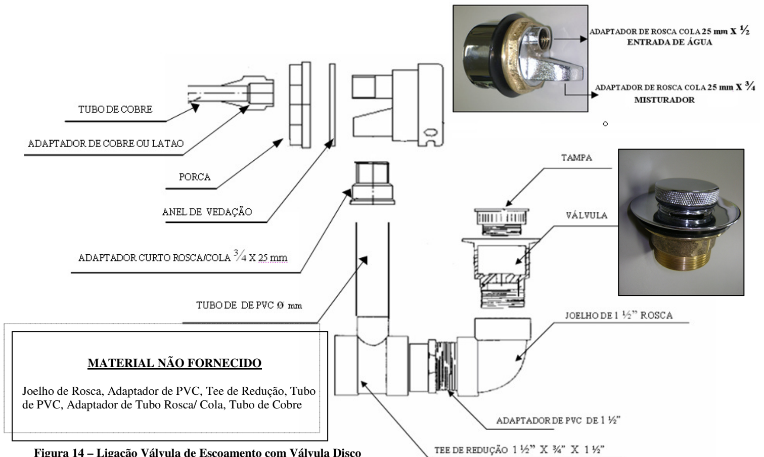
Figura 14 – Ligação Válvula de Escoamento com Válvula Disco
