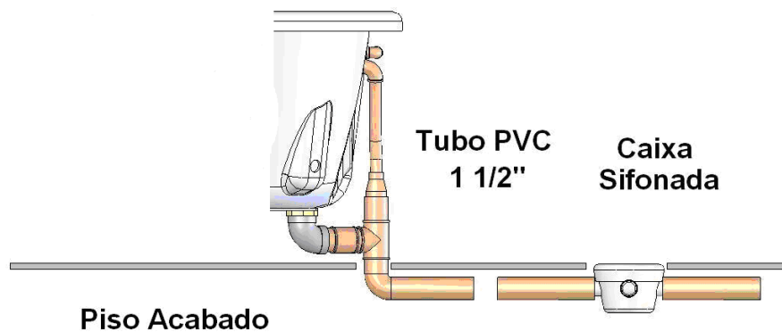
Figura 15 – Ligação da Válvula de Saída ao ponto de esgoto
