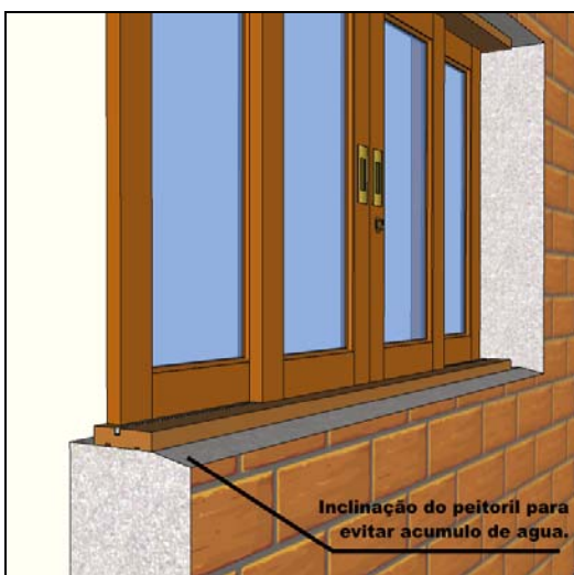
Figura 8 - Inclinação do peitoril da janela evita acúmulo de água.
