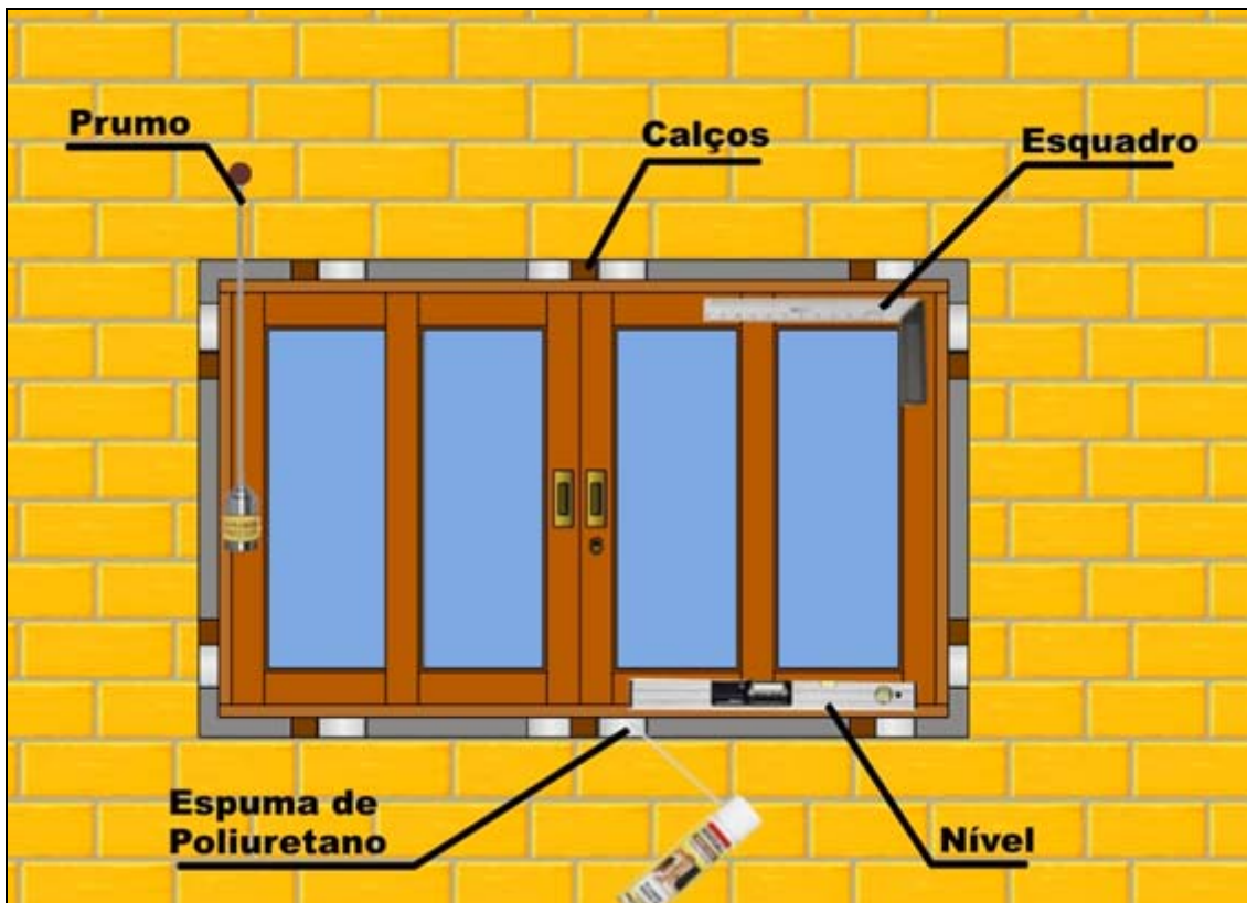
Figura 2 – Instalação da esquadria.
