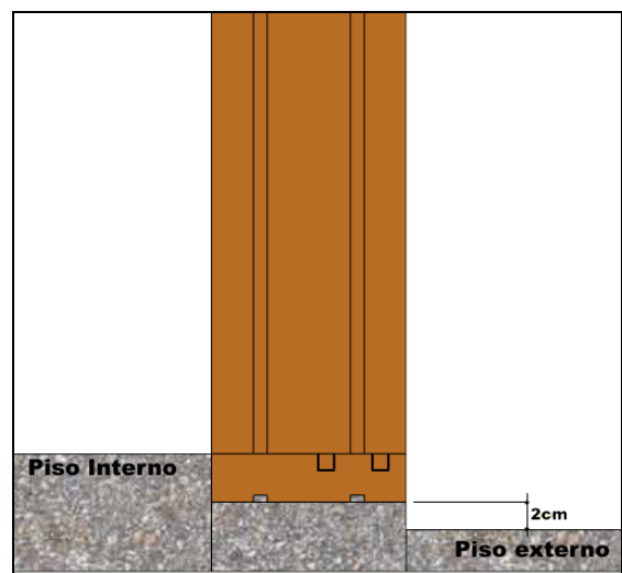
Figura 9 - Vãos de portas externas devem estar 2cm acima do piso externo.
