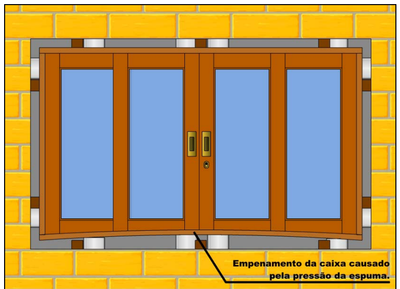
Figura 4 – Empenamento da esquadria causado pela pressão da espuma.
