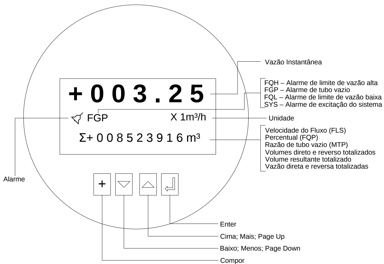
Figura 1 – Display e Botões do Hidrômetro
