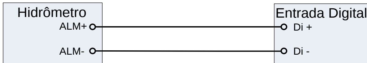
Figura 6 – Ligação da saída de alarme
