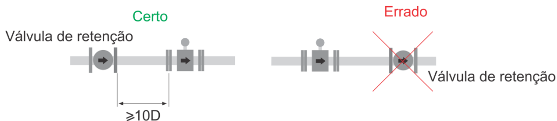
Figura 8 – A válvula de retenção deverá ser instalada antes do hidrômetro
