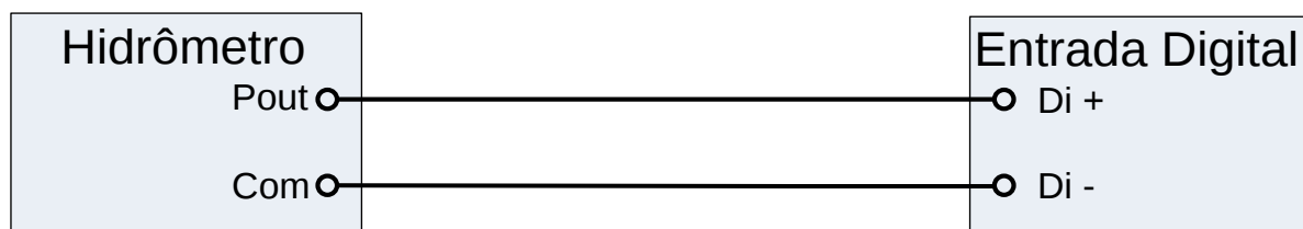
Figura 4 – Ligação da saída em pulsos/frequência para vazão totalizada
