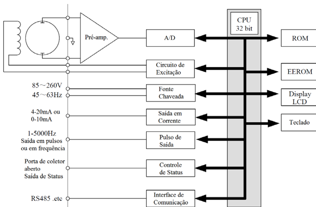
Figura 3 – Estrutura do conversor
