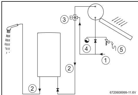
Fig. 20 Instalação solar
