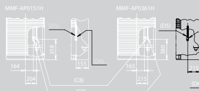
Posição da tubagem de refrigerante
