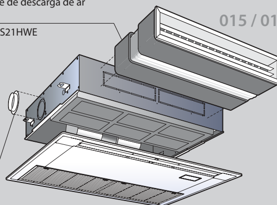
Grelha de 4 vias RBC-US21PGE
