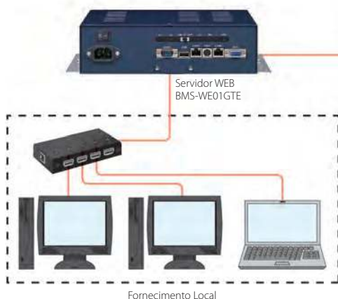
Diagrama de ligações para até 256 UIs
