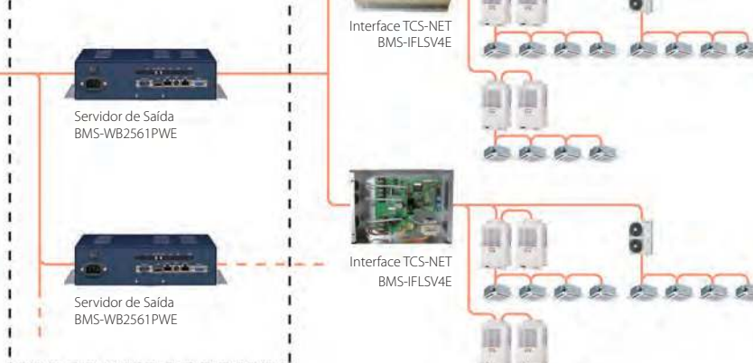
Diagrama de ligações até 256 UIs
