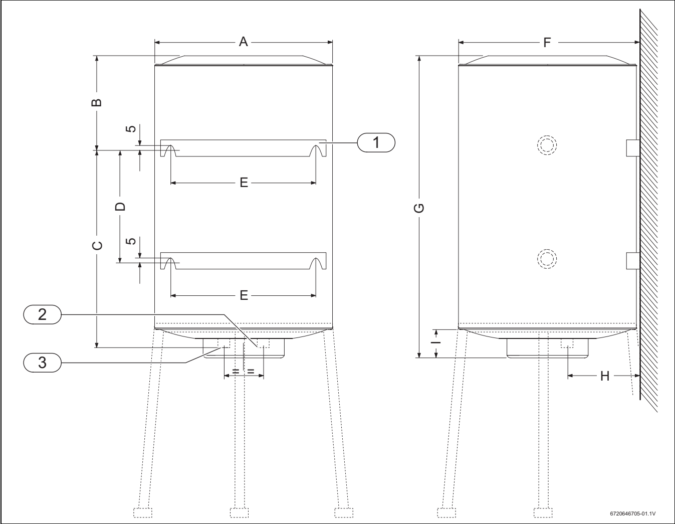
Fig. 2 Dimensões em mm (HS150/200-2...)
