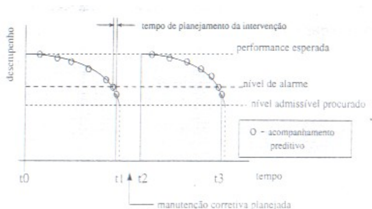
fig. 03 - Gráfico ilustrativo da manutenção preditiva.
