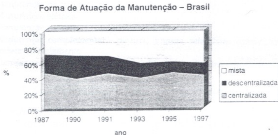
Fig. 5.6 - Evolução das Formas e Atuação da Manutenção no Brasil.
