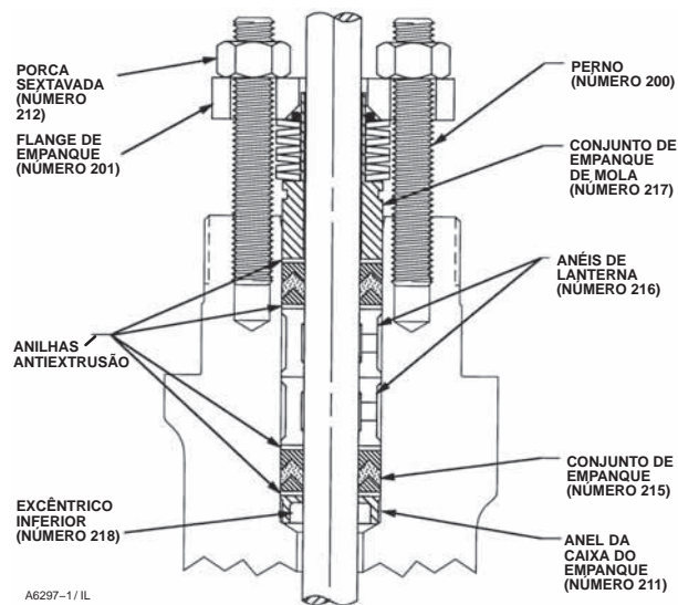
Figura 18. Sistema de Empanque Típico ENVIROSEAL com Empanque de PTFE da Fisher
