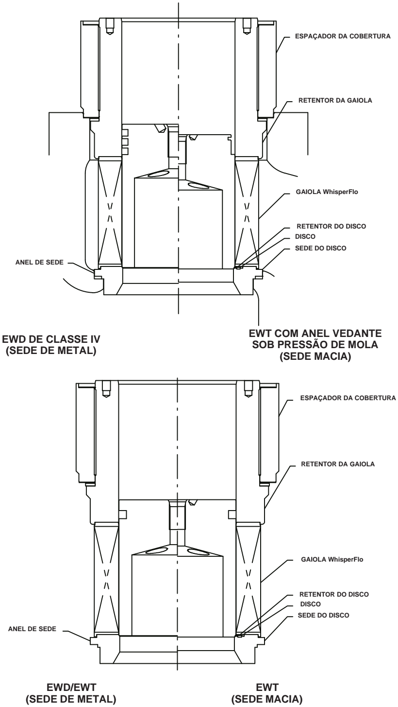
Figura 29. Internos Típicos WhisperFlo da Fisher
