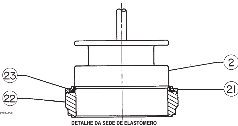
Figura 23. Válvula EWS da Fisher até NPS 12 x 6
