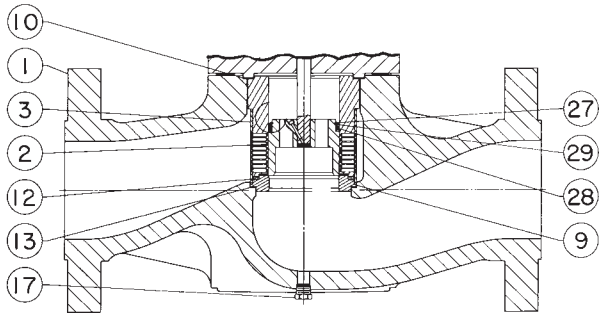
DETALHE DA JUNTA DA VÁLVULA NPS 8 x 6 CL900 COM BUJÃO DE DRENAGEM OPCIONAL
