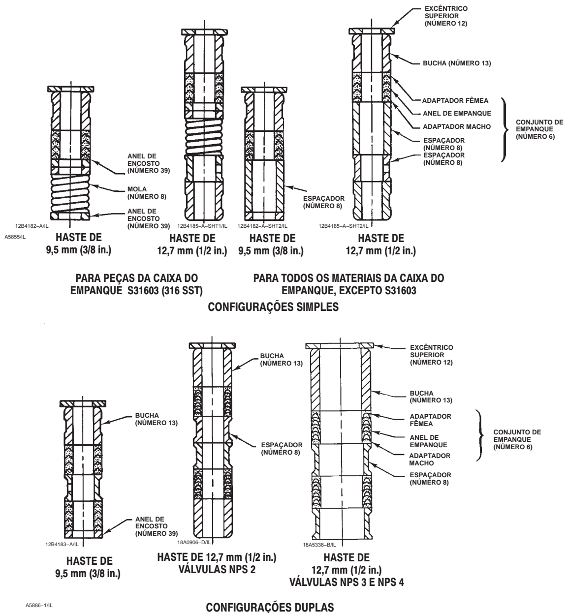
Figura 15. Configurações do Empanque de PTFE para Coberturas de Vedação de Foles ENVIROSEAL da Fisher
