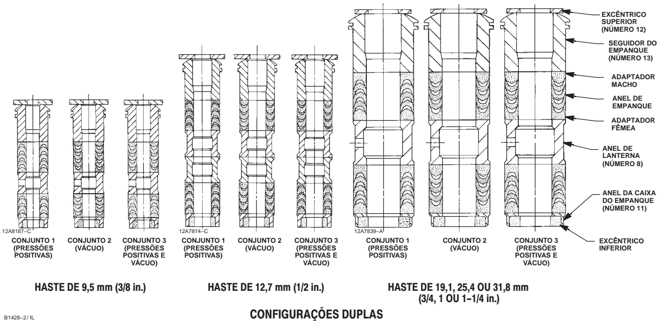
Figura 4. Configurações de Empanques de Anel em V de PTFE
