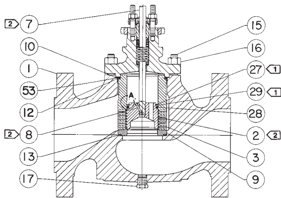
VÁLVULAS NPS 4 x 2 A 12 x 6 COM BUJÃO DE DRENAGEM OPCIONAL
