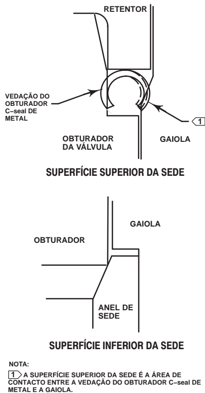
Figura 13. Superfícies Inferior (Obturador da Válvula para Anel de Sede) e Superior (Vedação do Obturador C-seal para Gaiola) da Sede
