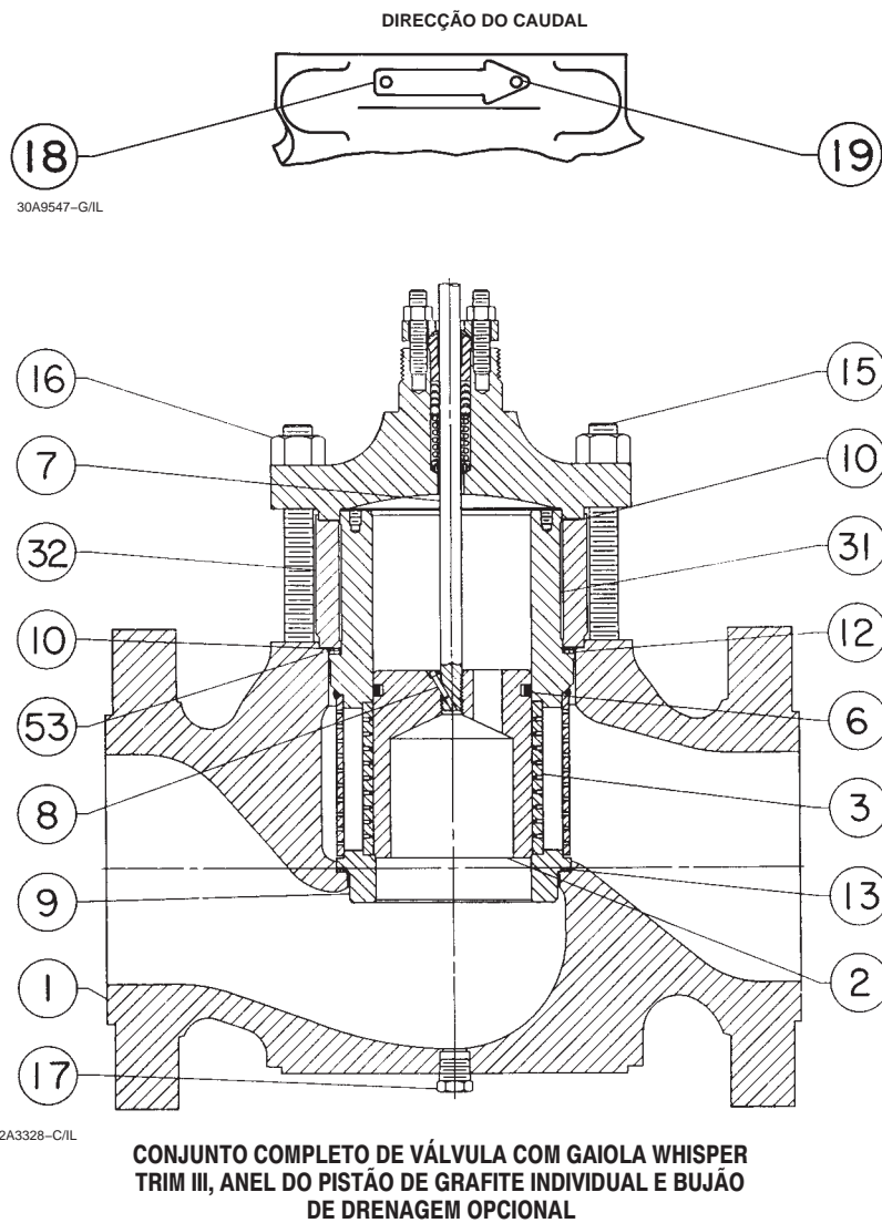
Figura 28. Válvula Típica EWD da Fisher com Gaiola Whisper Trim III
