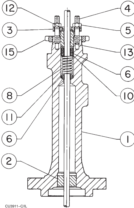
COBERTURA DE PROLONGAMENTO TIPO 1 OU 2
