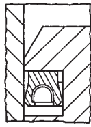
VISTA A VÁLVULAS NPS 8 x 6 A 12 x 6
