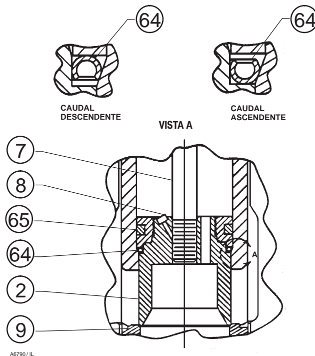
Figura 9. EWD da Fisher com Internos C-seal
