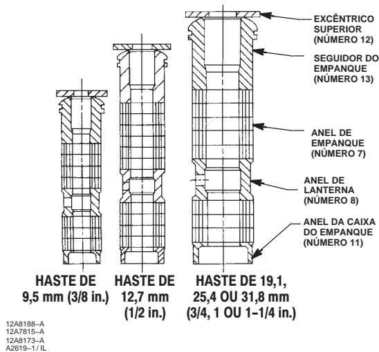
Figura 5. Detalhe de Configurações de Empanque de PTFE/Composição
