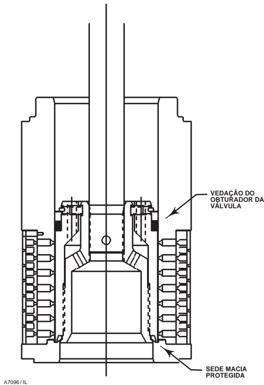
Figura 8. Internos TSO Equilibrados Típicos
