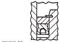
VISTA A VÁLVULAS NPS 4 x 2 A 8 x 4
