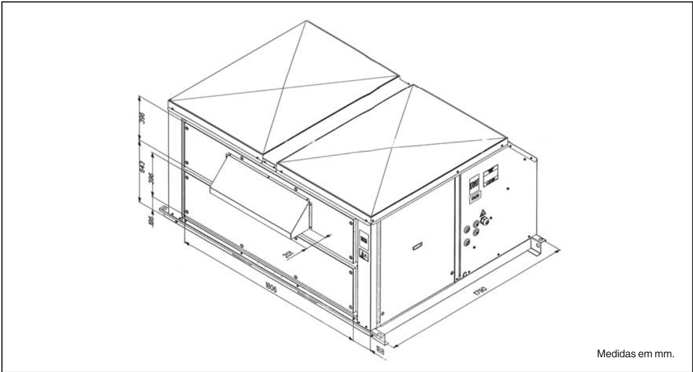
Figura 2b - Dimensões das unidades 40RT
