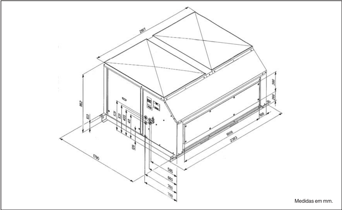
Figura 2a - Dimensões das unidades 40RT
