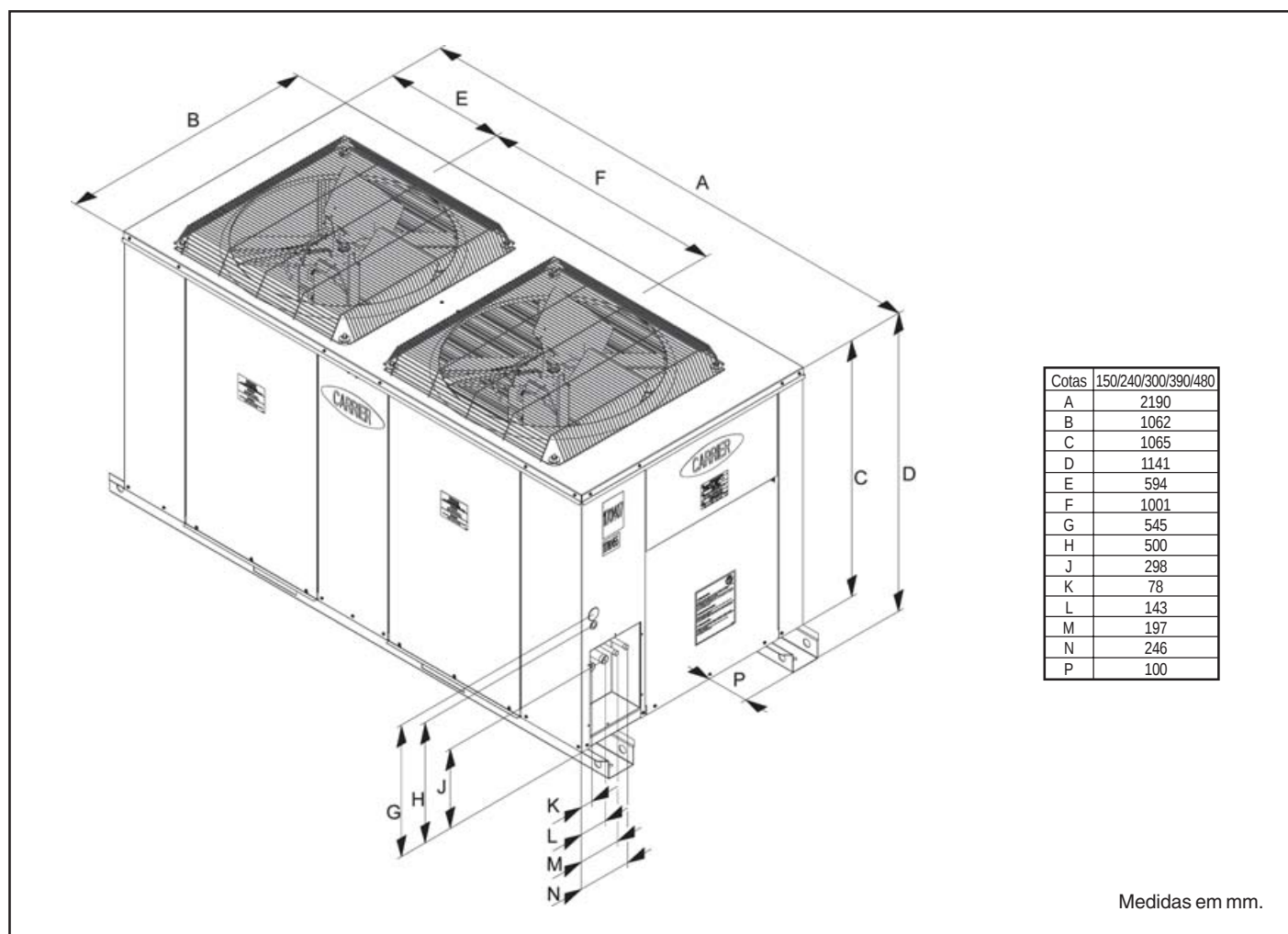
Fig. 2c - Dimensões da Unidade 38AB
