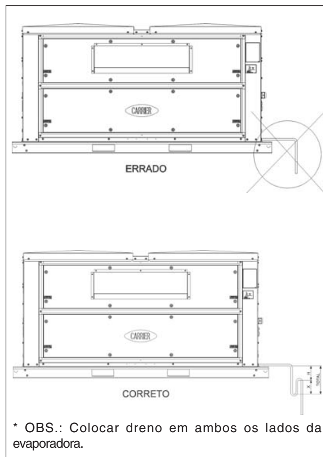
Figura 5 - Conexões para dreno
