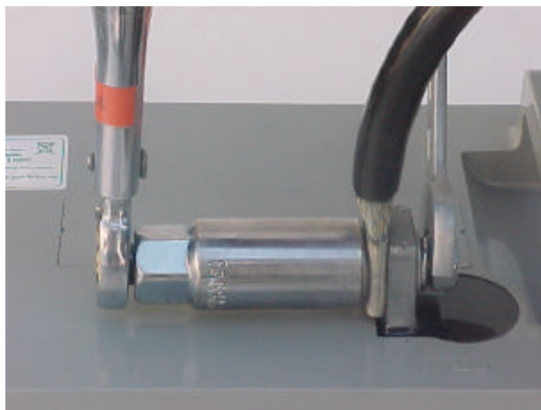
2 d – CONEXÃO FINAL COM TORQUIMETRO DE ESTALO
