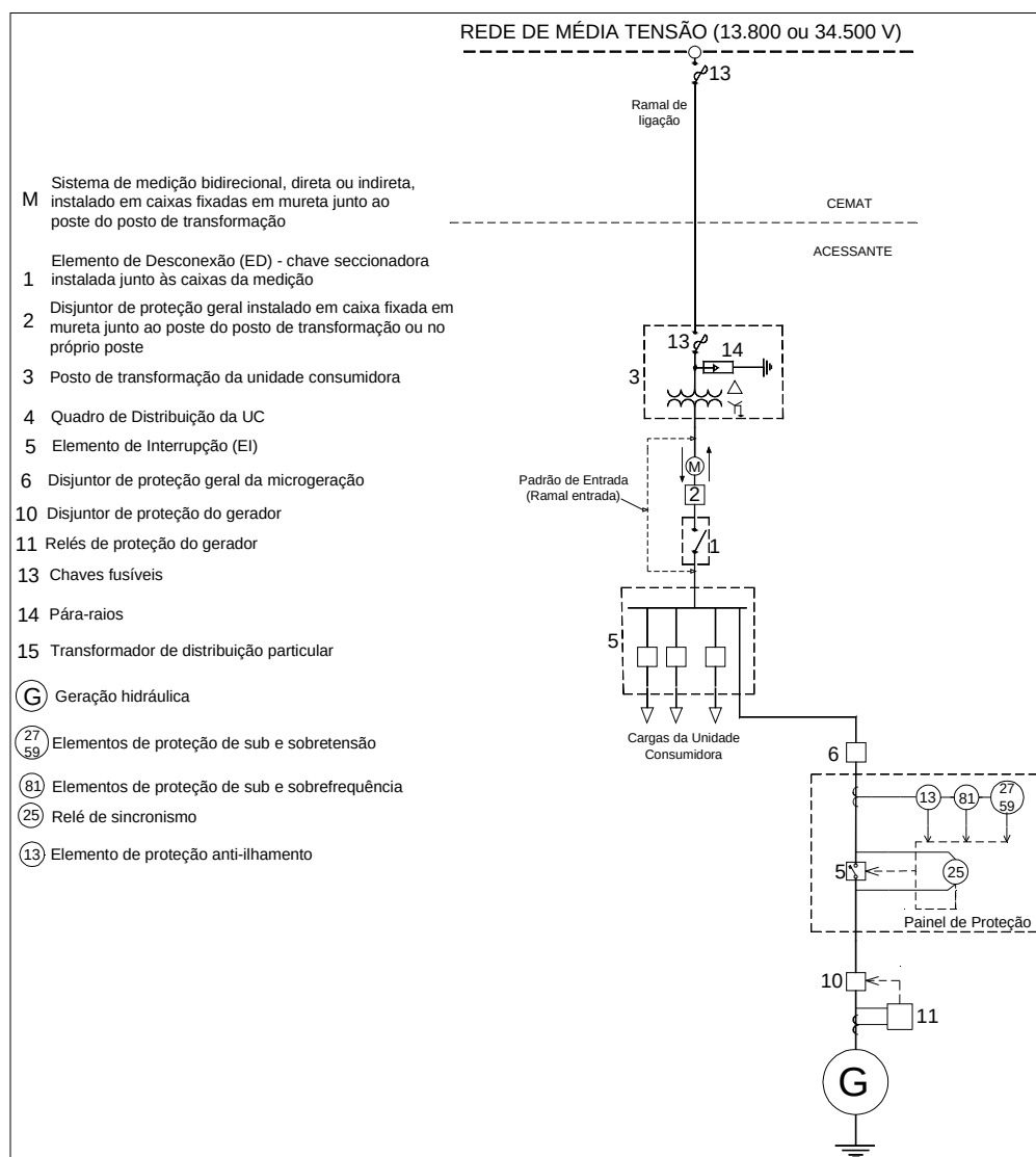
FIGURA 8 - Conexão de microgeração através de unidade consumidora do GA
