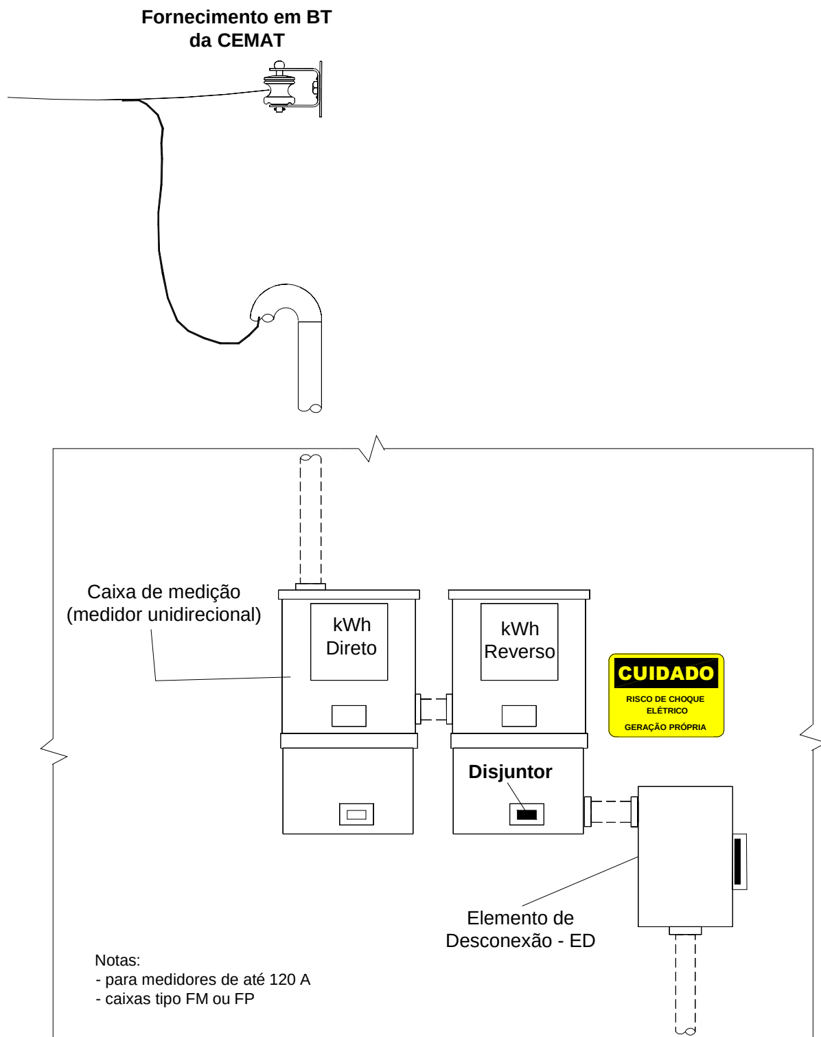
FIGURA 13 - Disposição do Elemento de Desconexão - ED - instalado junto à medição e proteção no padrão de entrada em muro ou mureta - com dois medidores unidirecionais
