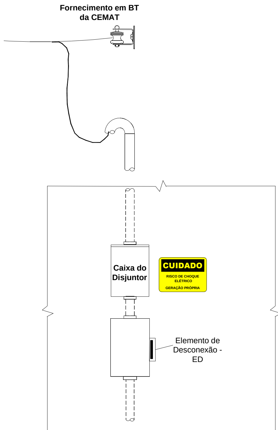
FIGURA 16 - Disposição do Elemento de Desconexão - ED - instalado junto à proteção no padrão de entrada em muro ou mureta - com a medição externa no poste da RD
