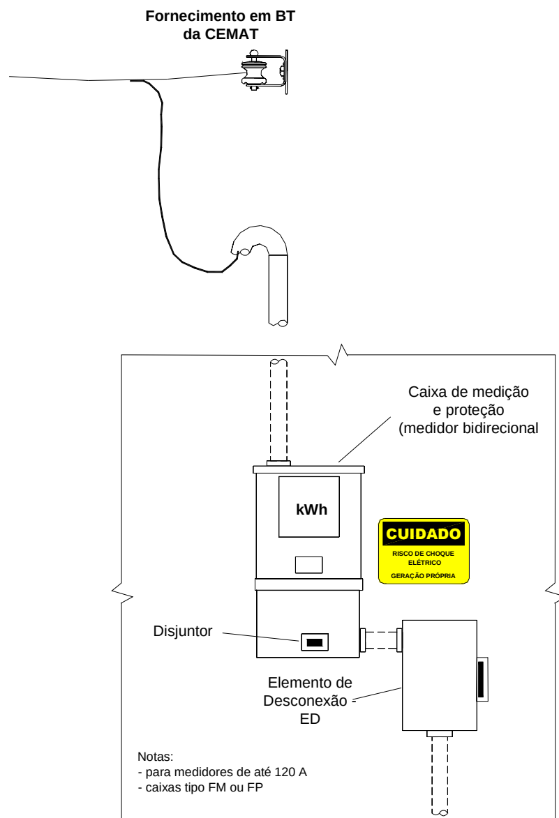
FIGURA 12 - Disposição do Elemento de Desconexão - ED - instalado junto à medição e proteção no padrão de entrada em muro ou mureta - com medidor Bidirecional
