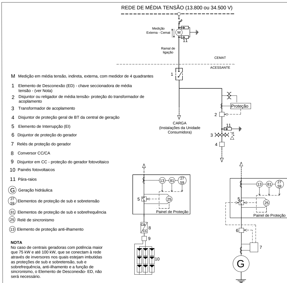
FIGURA 1 - Conexão de geração distribuída com potência instalada de 75,1 a 500 kW, através de unidade consumidora do GA
