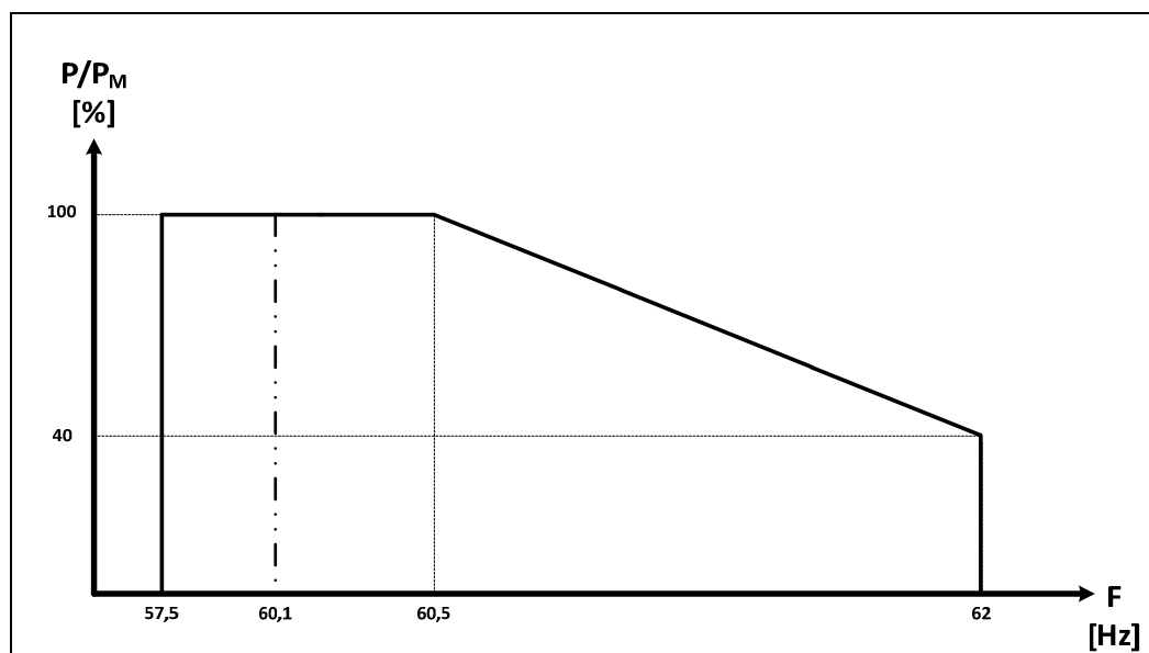
FIGURA 3 – Curva de operação do sistema de geração distribuída em função da frequência da rede para desconexão por sub e sobrefrequência.
