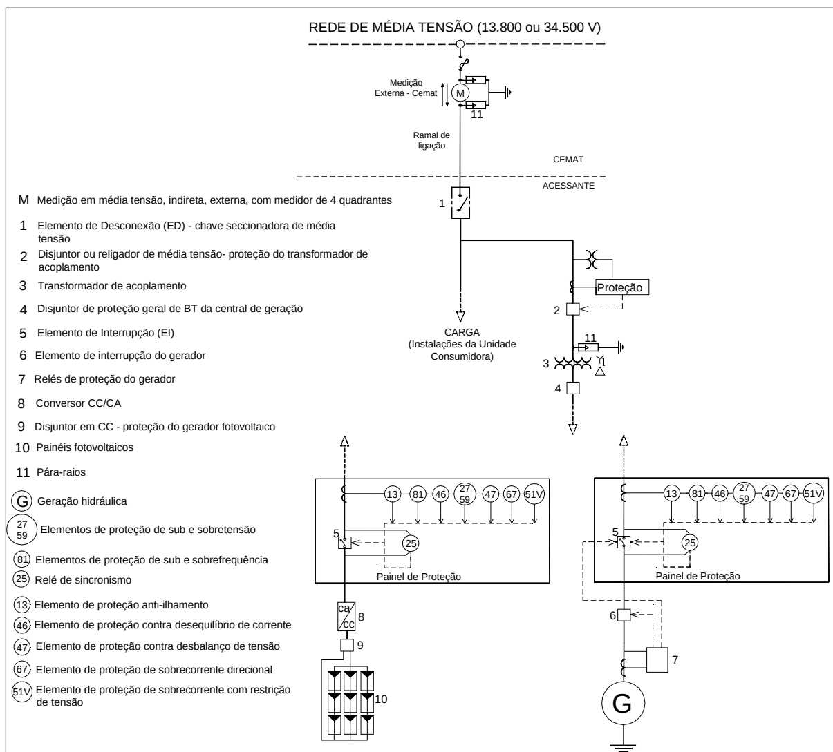
FIGURA 2 - Conexão de geração distribuída com potência instalada de 501 a 1000 kW, através de unidade consumidora do GA
