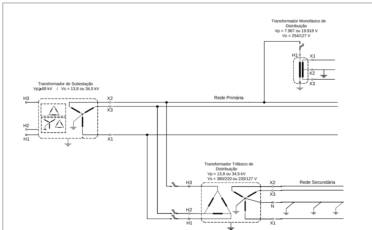
FIGURA 5 - Diagrama simplificado do sistema de distribuição da CEMAT
