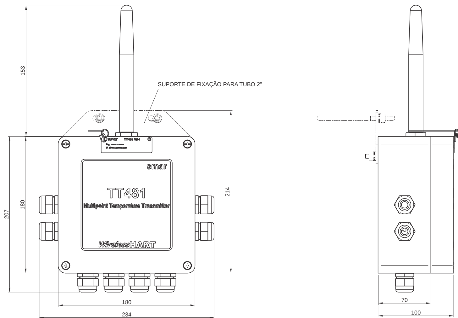
Figura 1.1 (b) - Desenho Dimensional - TT481 WirelessHART™ com 8 Canais
