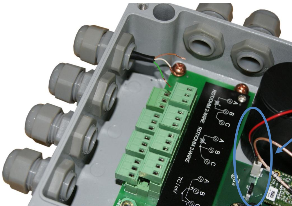
Figura 1.3 – Conexão do Módulo de Baterias à Placa Eletrônica
