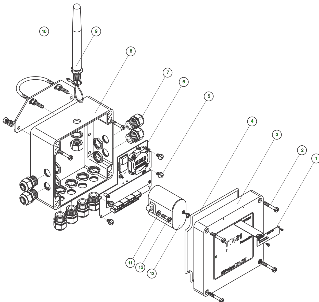
Figura 3.1 (b) – Desenho Explodido do TT481 WirelessHART™ com 8 Canais
