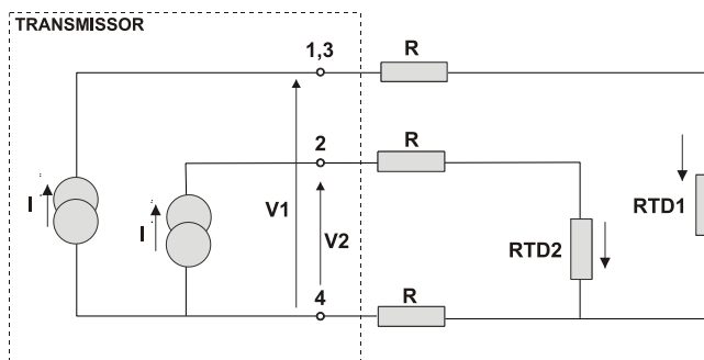
Figura 2.4 - Conexão Diferencial
