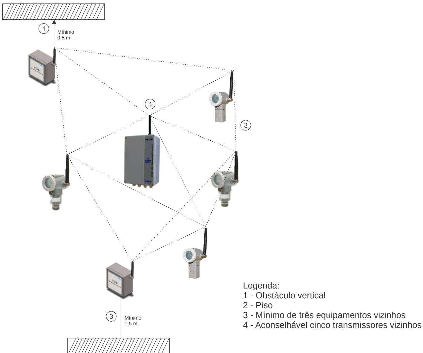
Figura 1.2 – Esquema de Ligação para Transmissores Wireless
