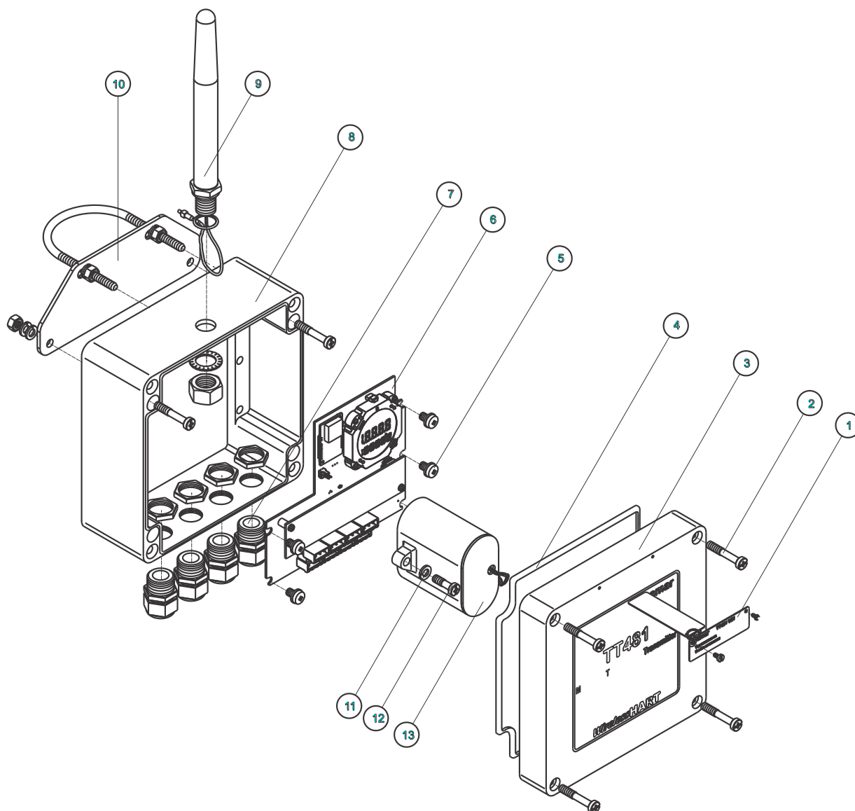
Figura 3.1 (a) – Desenho Explodido do TT481 WirelessHART™ com 4 Canais
