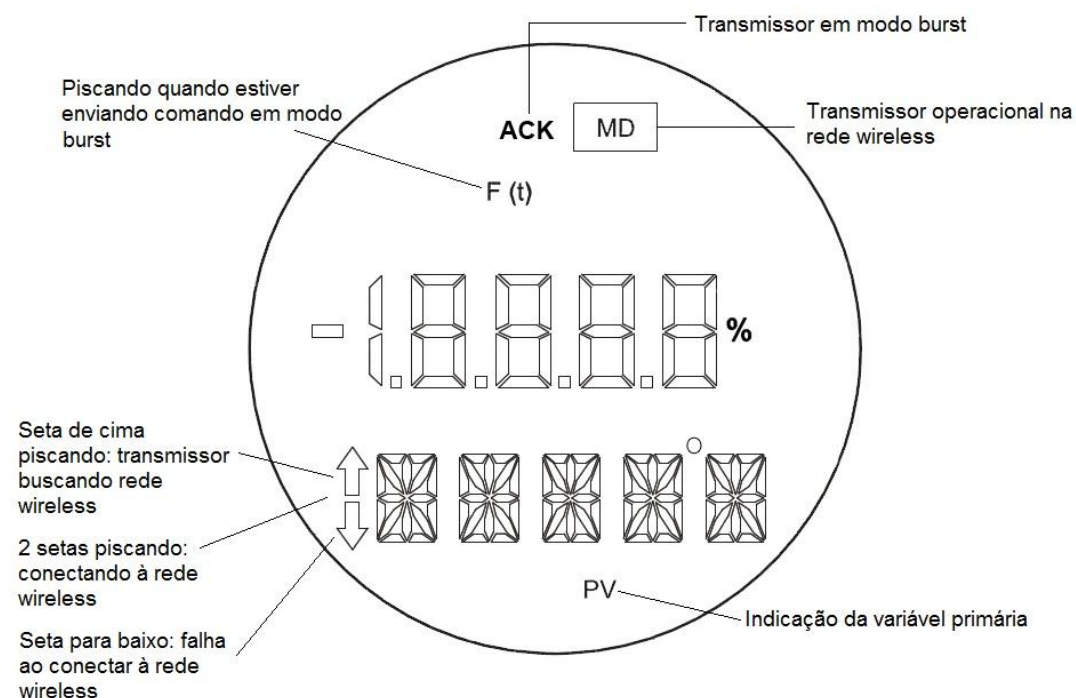
Figura 2.5 – Display
