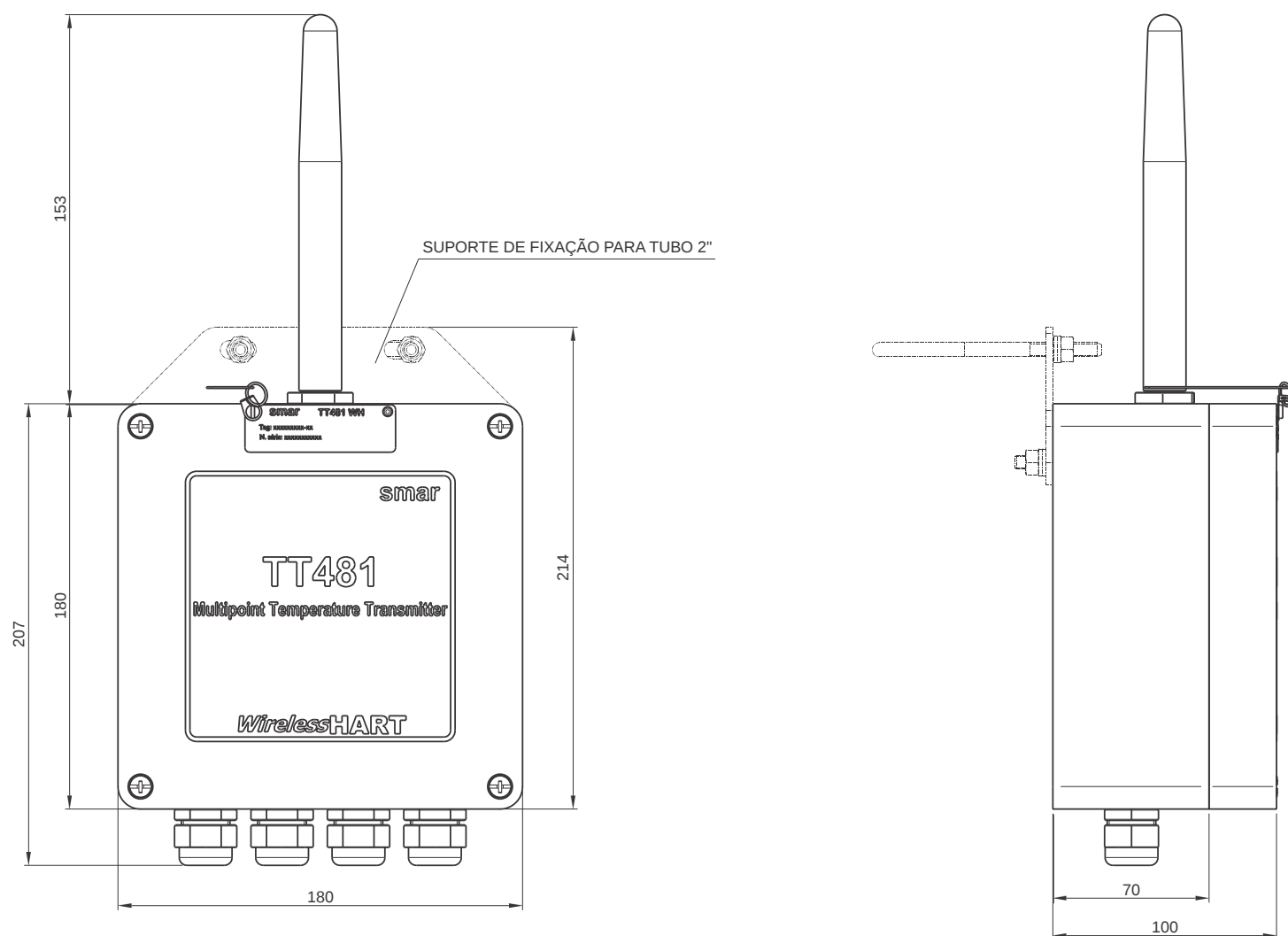
Figura 1.1 (a) - Desenho Dimensional - TT481 WirelessHART™ com 4 Canais
