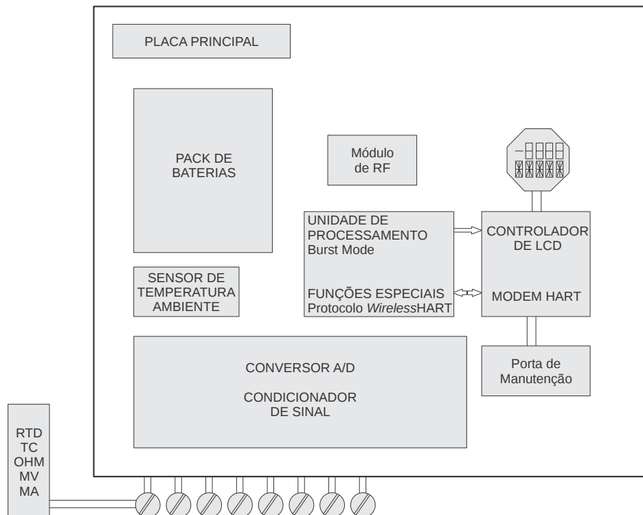
Figura 2.1 - Diagrama de Bloco do TT481 WirelessHART™
