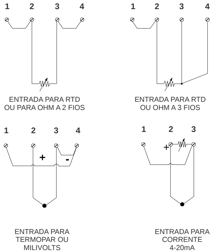
Figura 1.5 - Ligação dos Sensores
