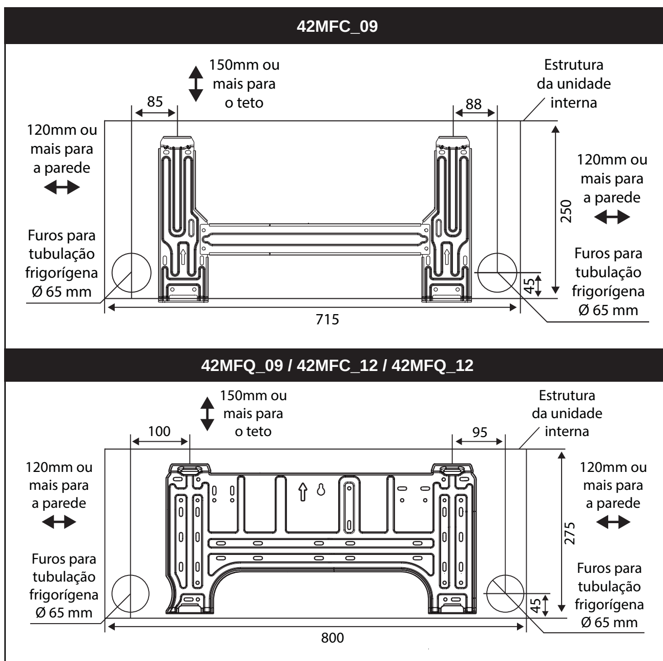
FIG. 20-A - PLACAS DE MONTAGEM
