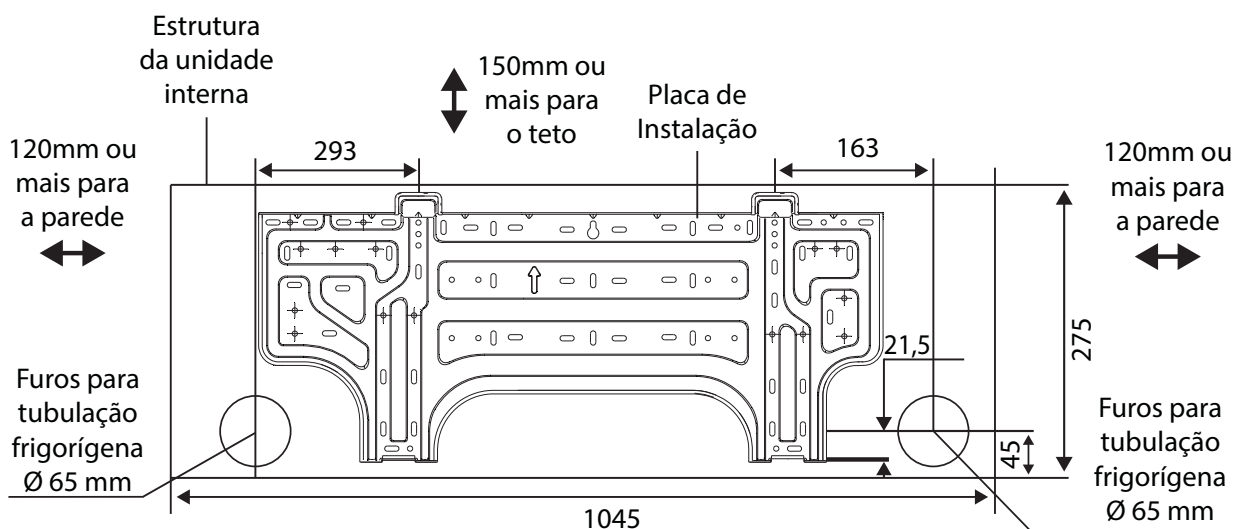
FIG. 20-B - PLACAS DE MONTAGEM
