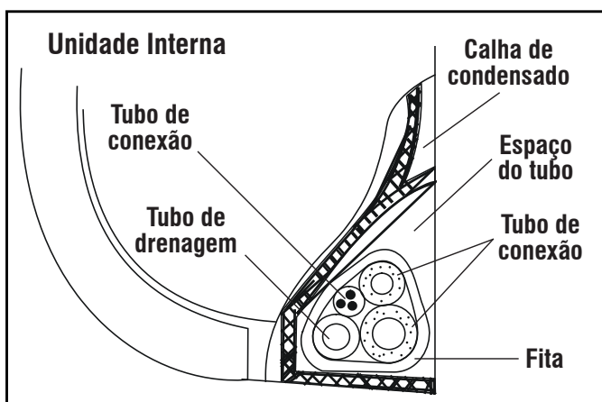
FIG. 16 - TUBO DE CONEXÕES
