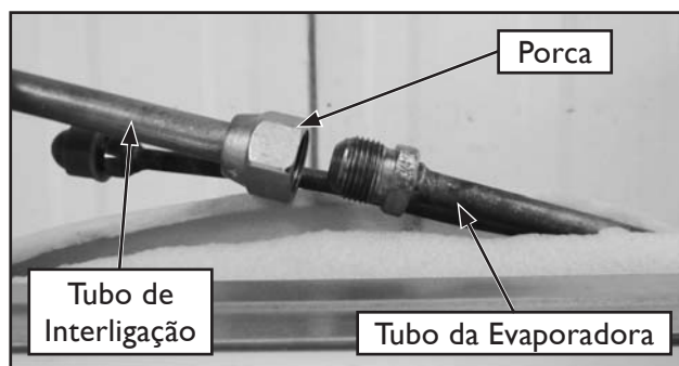
FIG. 33 - CONEXÃO DA LINHA DE SUÇÃO
