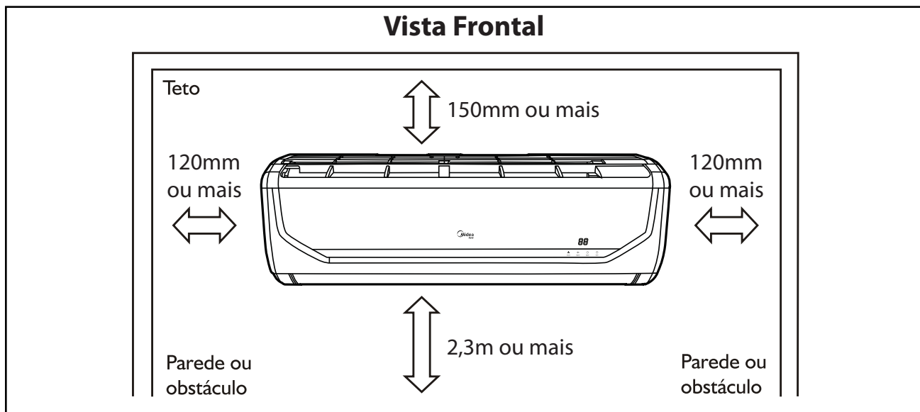
FIG. 13 - ESPAÇAMENTOS MÍNIMOS RECOMENDADOS
