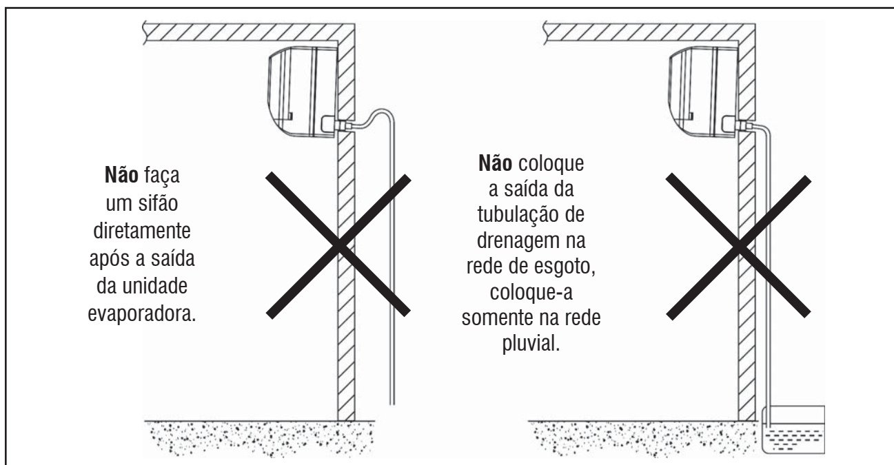
FIG. 14 - SITUAÇÕES DE DRENAGEM INEFICAZ
