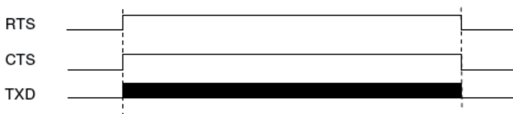
Figura 7-4. Timing dos Sinais RTS, CTS e TXD
