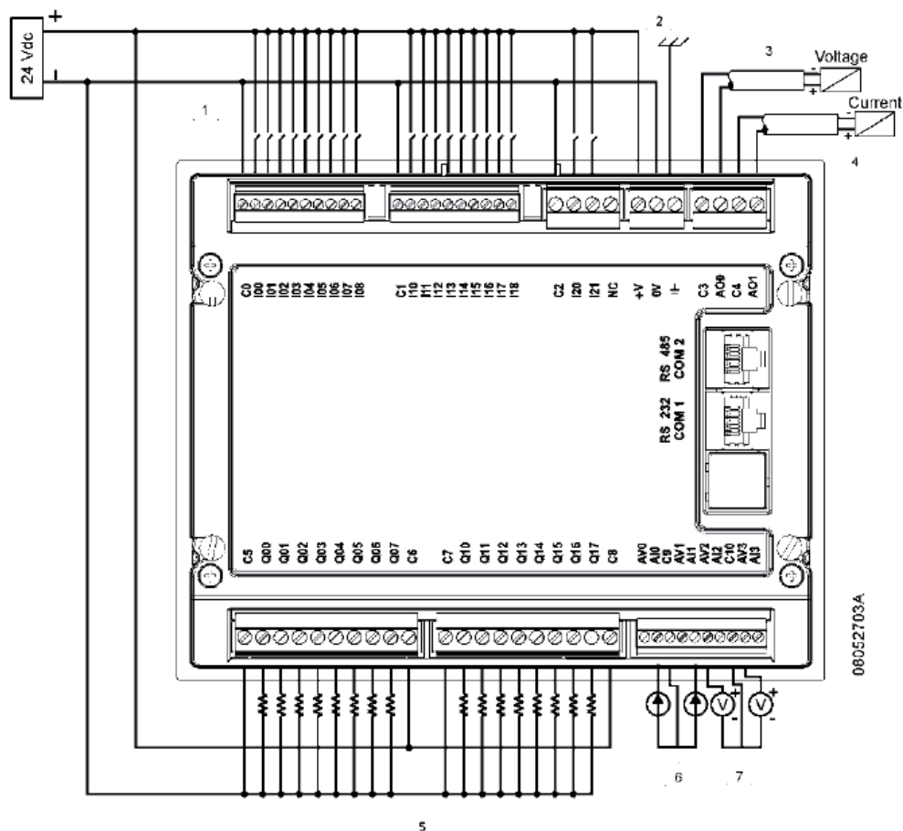
Figura 4-1. Exemplo de Ligação CPS-4000
