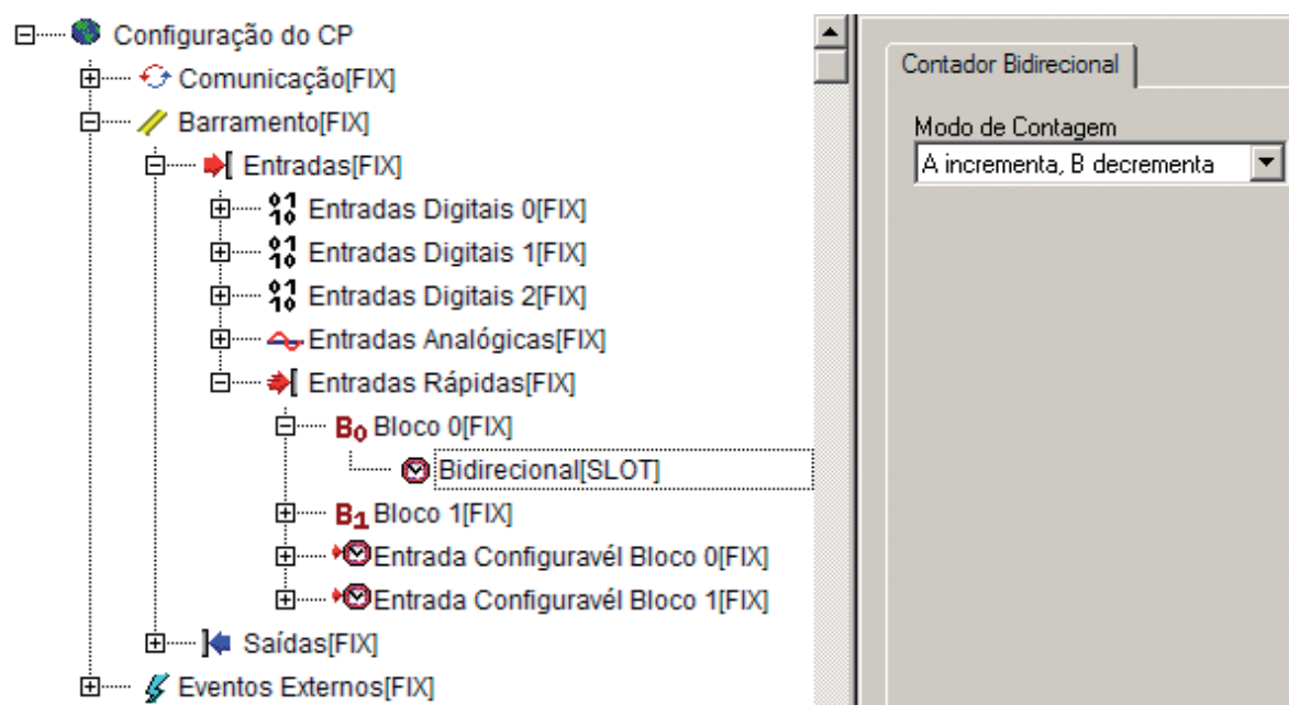
Figura 3-9. Contador Bidirecional
