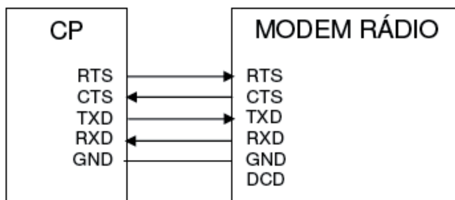
Figura 7-2. Conexão do CP com um Modem Rádio
