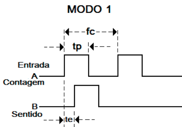
Figura 3-7. Bidirecional Modo 1
