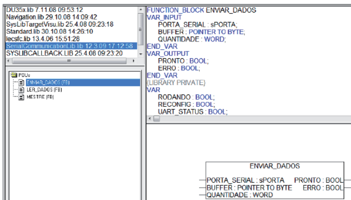
Figura 3-38. Biblioteca de comunicação carregada
