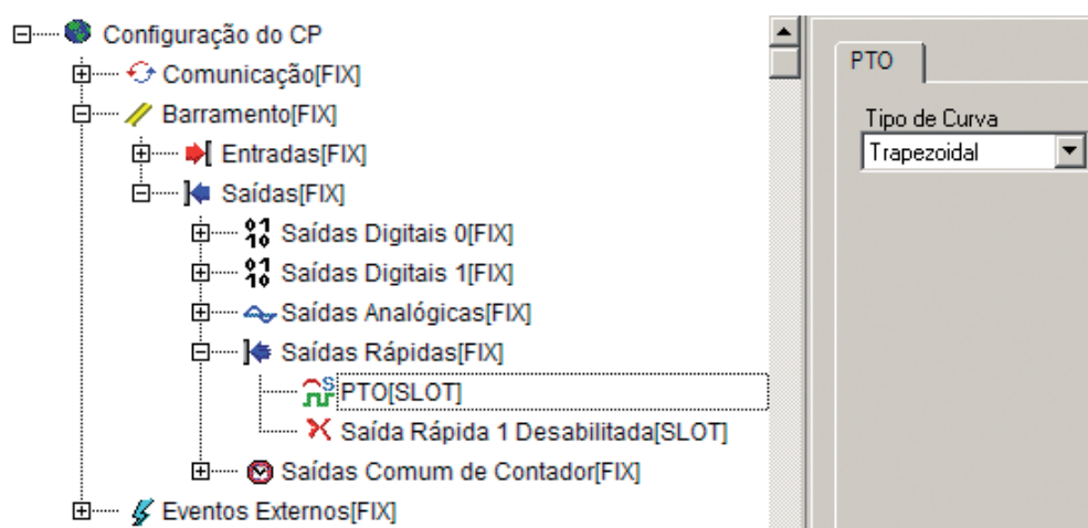
Figura 3-19. PTO
