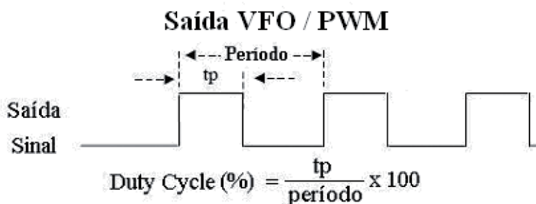
Figura 3-20. VFO/PWM
