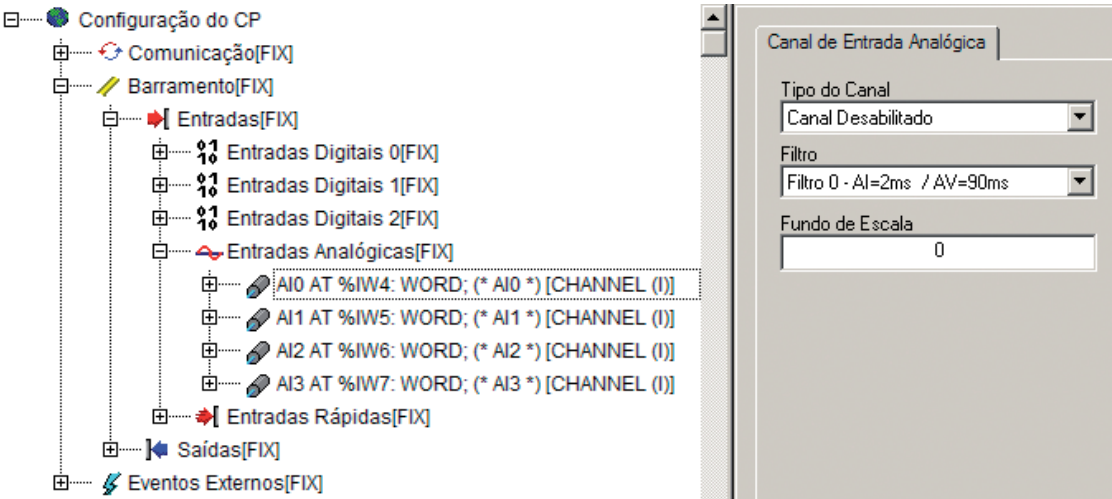
Figura 3-3. Entradas Analógicas
