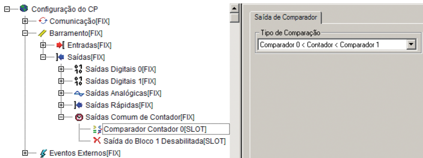
Figura 3-23. Configurando a saída comum de contador
