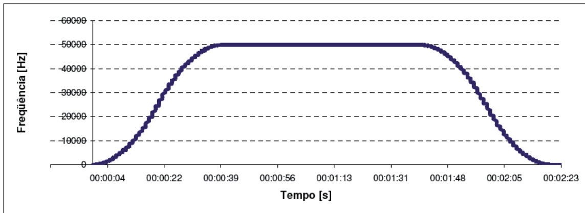
Figura 3-17. Gráfico gerado por uma saída PTO utilizando o perfil do tipo S
