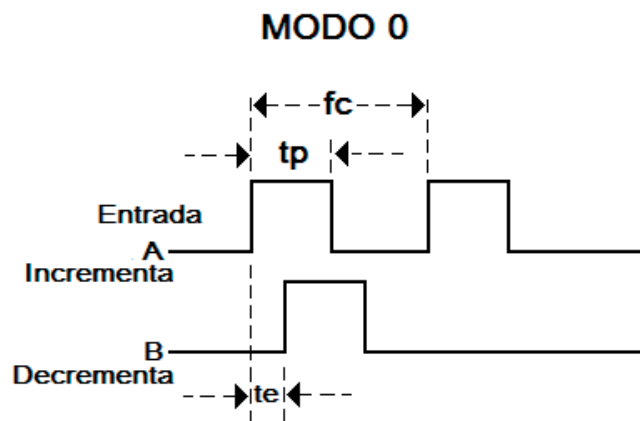
Figura 3-6. Bidirecional Modo 0
