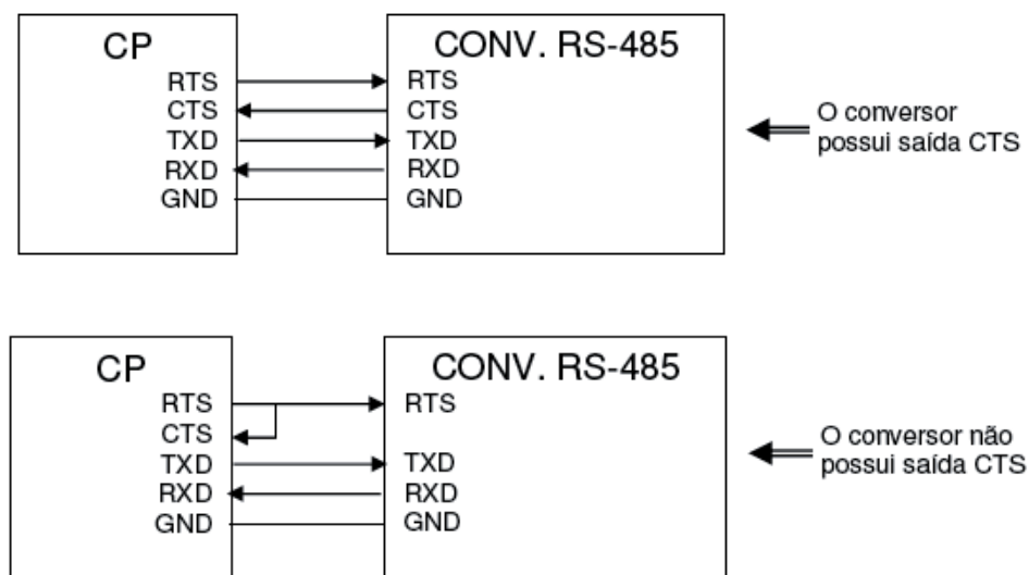
Figura 7-3. Conexão do CP com um Conversor RS-485
