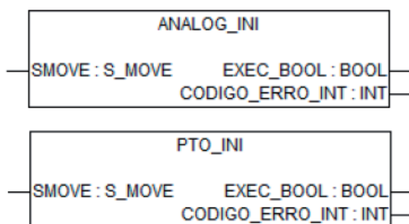
Figura 3-24. Blocos Funcionais ANALOG_INI e PTO_INI
