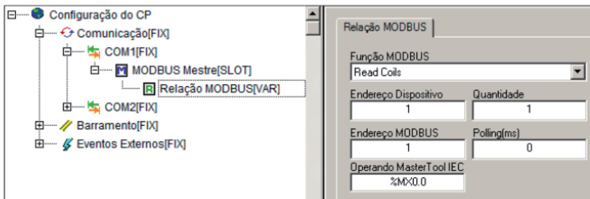
Figura 3-31. Relação MODBUS
