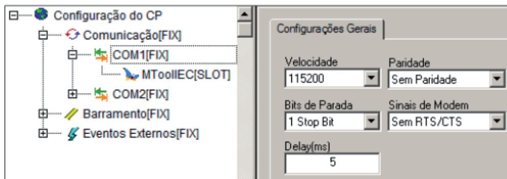
Figura 3-29. Configurando COM1
