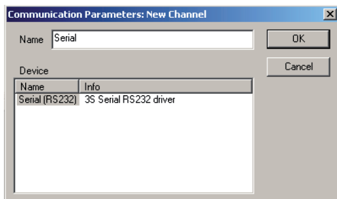
Figura 5-1. Nova Conexão
