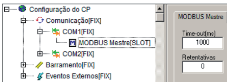
Figura 3-30. MODBUS Mestre
