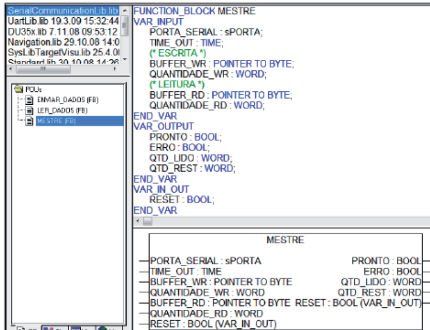
Figura 3-41. Detalhamento da declaração das entradas e saídas do bloco funcional MESTRE
