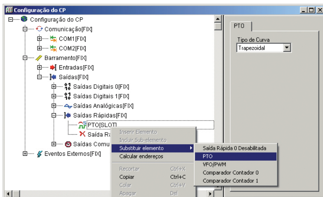
Figura 3-14. Saídas Rápidas
