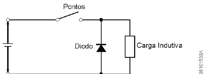
Figura 4-4. Circuito de Proteção das Saídas Digitais
