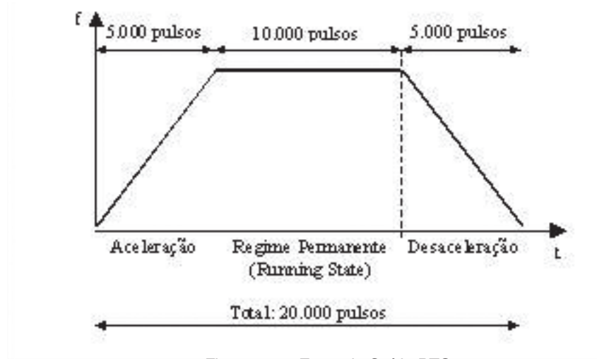
Figura 3-15. Exemplo Saída PTO
