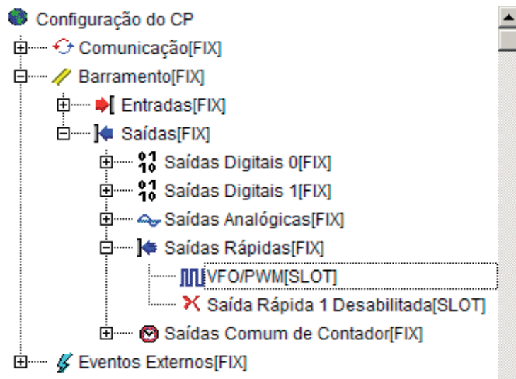
Figura 3-21. Configurando para VFO/PWM
