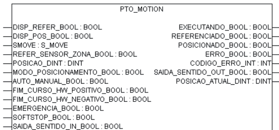
Figura 3-27. Bloco Funcional PTO_MOTION
