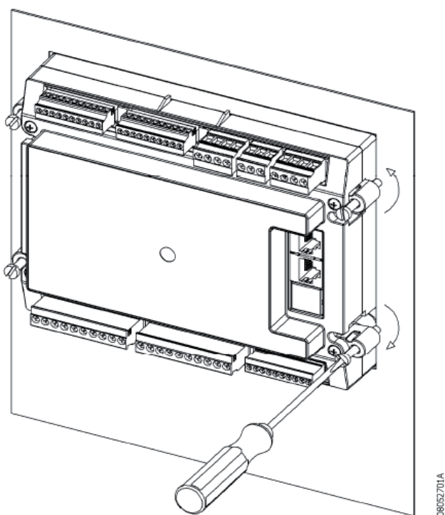
Figura 4-8. Fixação Mecânica
