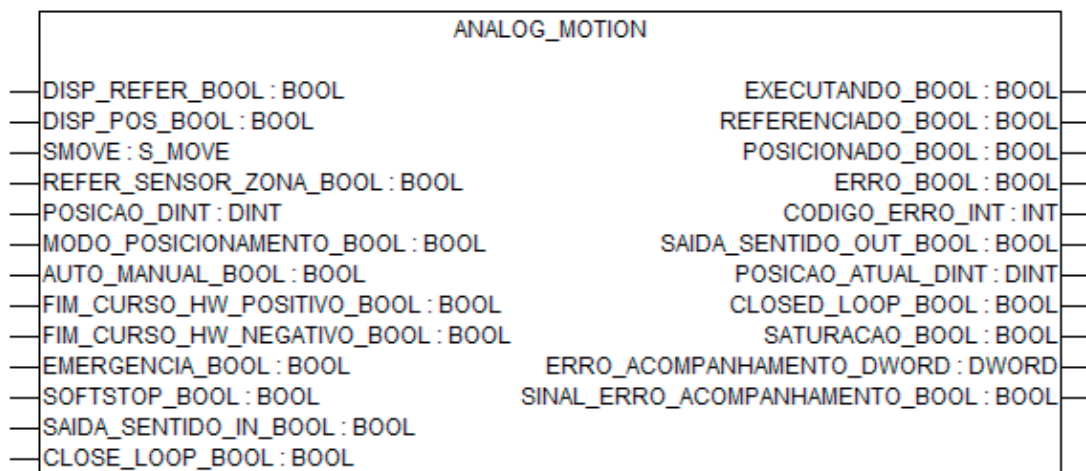
Figura 3-28. Bloco Funcional ANALOG_MOTION
