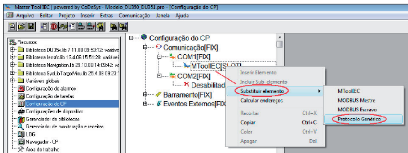
Figura 3-34. Procedimento de substituição de elemento em uma porta de comunicação
