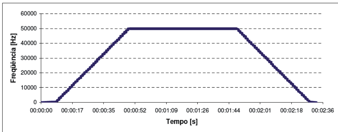
Figura 3-16. Gráfico gerado por uma saída PTO utilizando o perfil do tipo Trapezoidal
