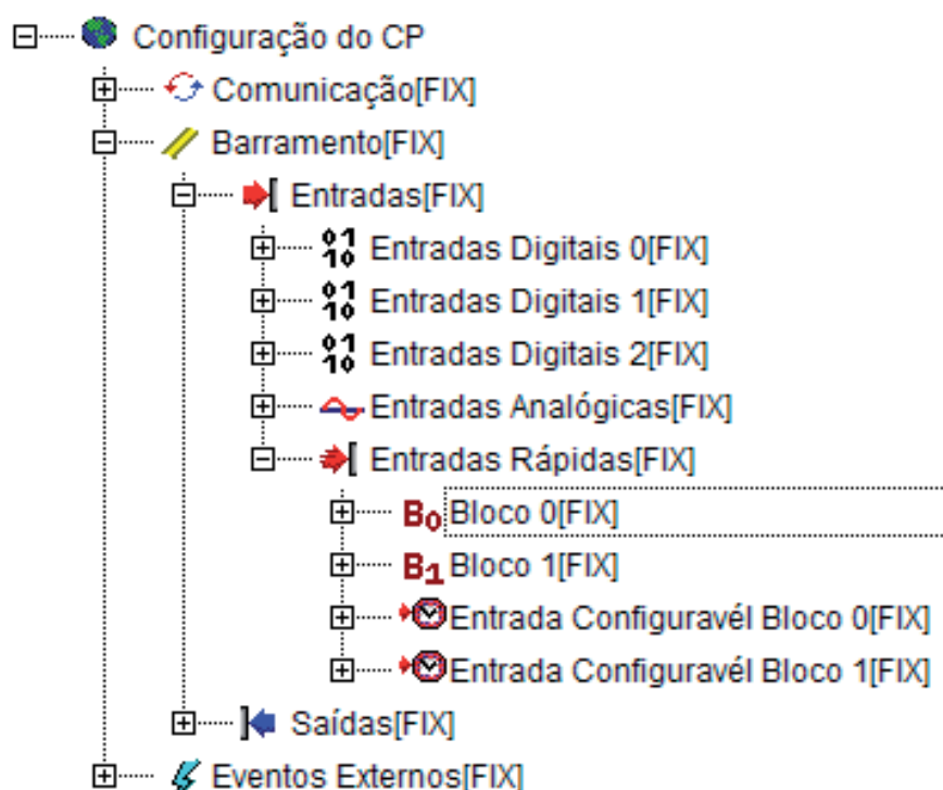
Figura 3-4. Entradas Rápidas
