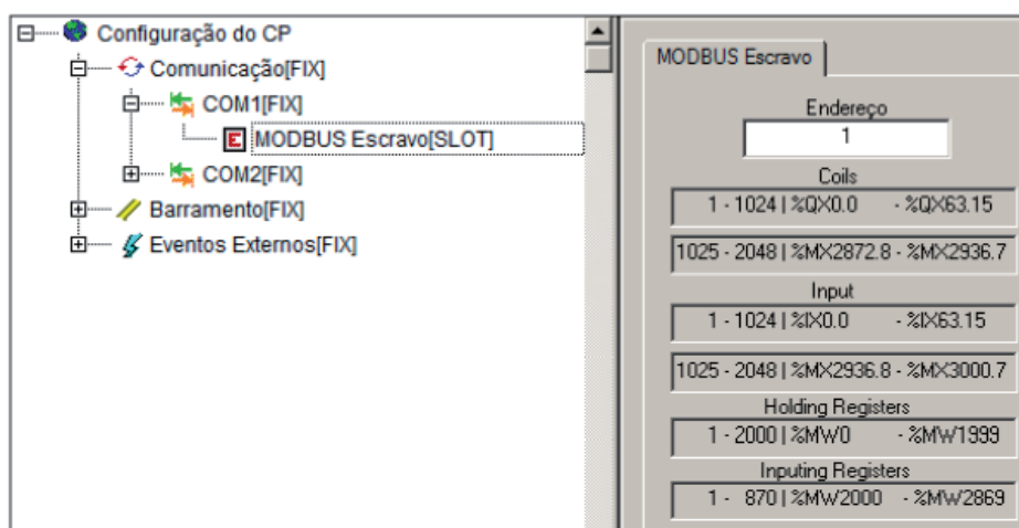
Figura 3-32. Relação MODBUS
