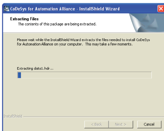
Figura 4-9. Extraíndo Arquivos
