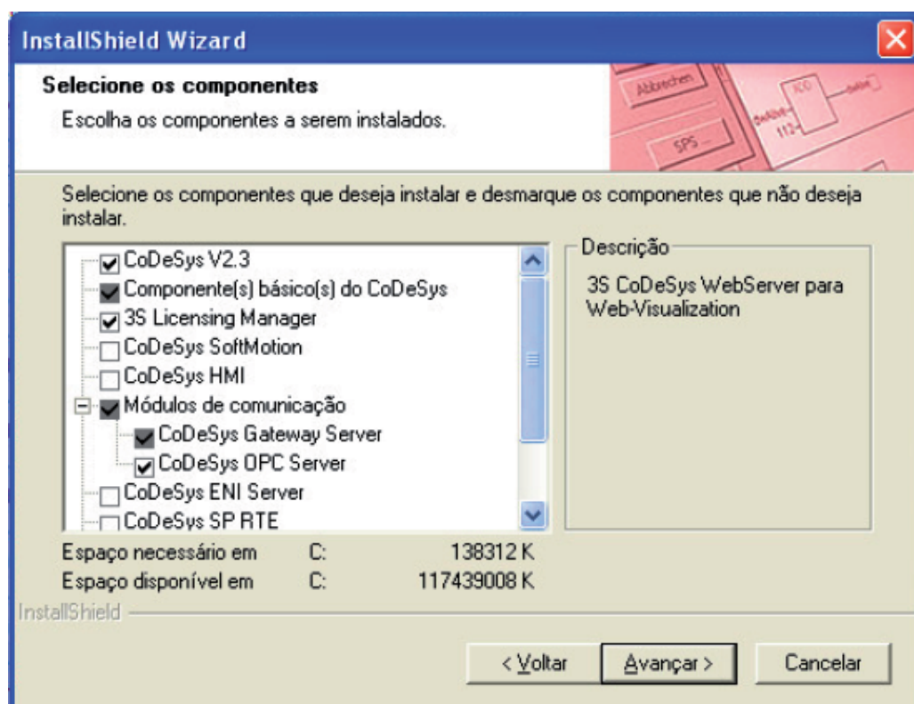
Figura 4-12. Componentes
