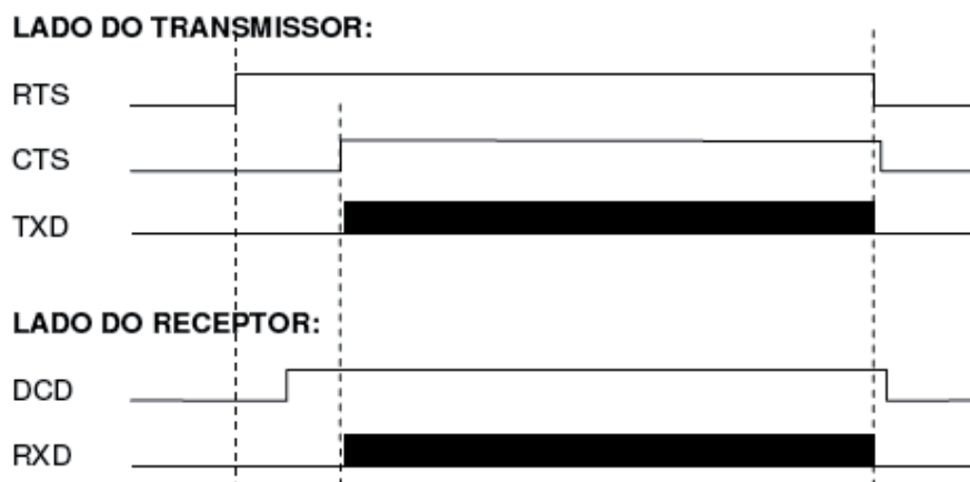
Figura 7-1. Timing dos Sinais RTS, CTS e TXD
