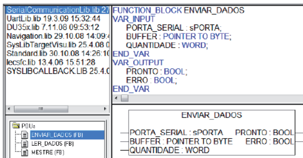
Figura 3-39. Detalhamento da declaração das entradas e saídas do bloco funcional ENVIAR_DADOS
