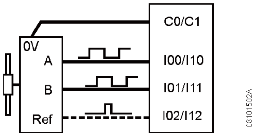
Figura 4-3. Exemplo de Ligação com Encoder
