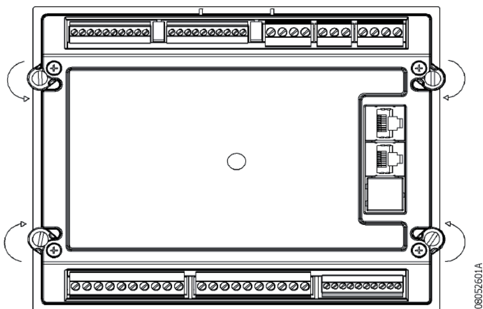
Figura 4-6. Presilhas Laterais
