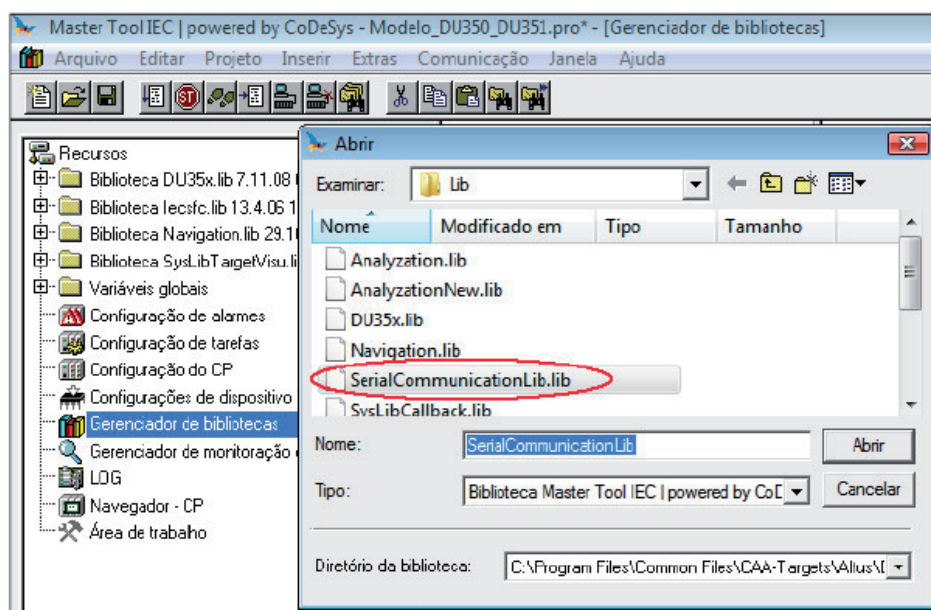
Figura 3-37. Inclusão da biblioteca de comunicação
