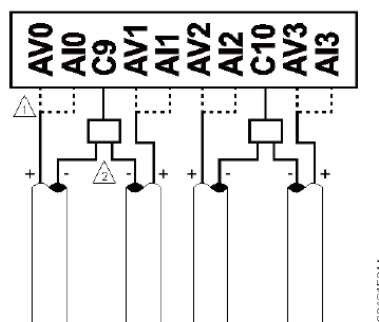
Figura 4-2. Ligação das Entradas Analógicas
