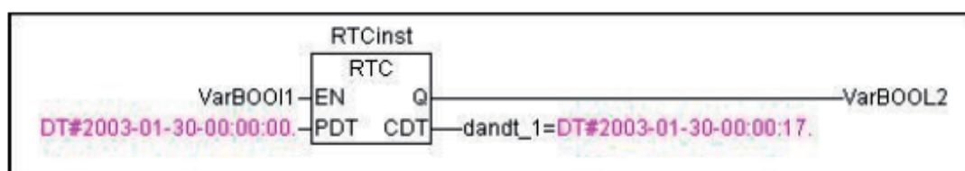
Figura 3-43. Bloco funcional RTC
