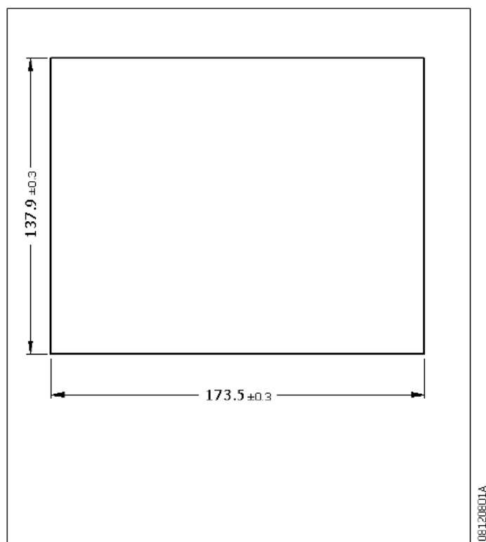
Figura 4-5. Corte do Painel para Instalação
