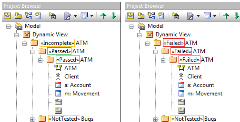
Figura 5.11: Explorador de Projetos com os estereótipos dos pacotes editados pelo FEUP-SBT-2.0.
