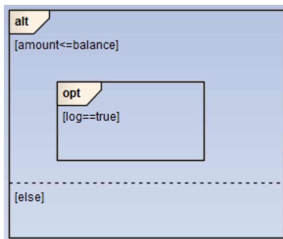
Figura B.4: Fragmentos combinados do exemplo "ATM" isolados.
