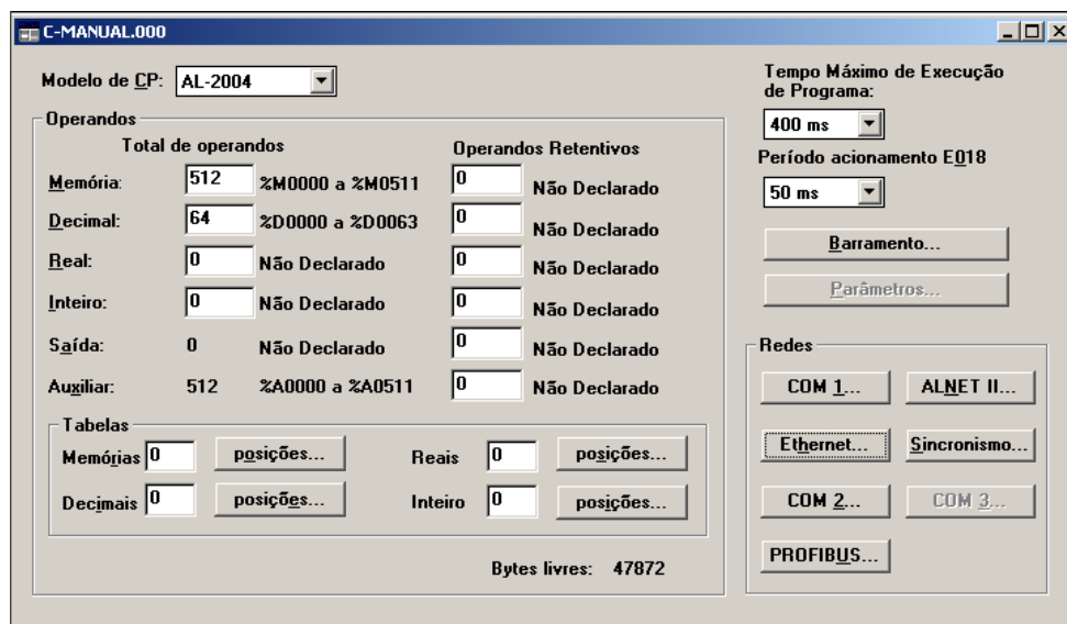
Figura 3-5. Configuração dos parâmetros Ethernet
