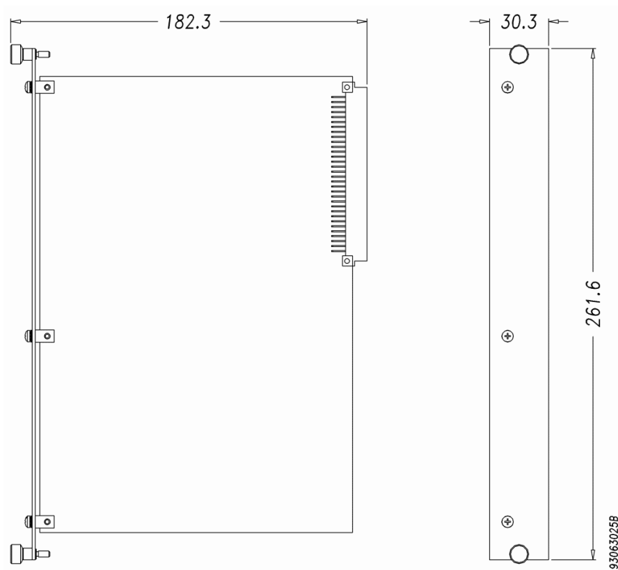
Figura 2-6. AL-3414 - Dimensões físicas
