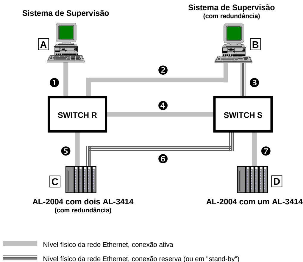
Figura 2-4. Rede de comunicação redundante
