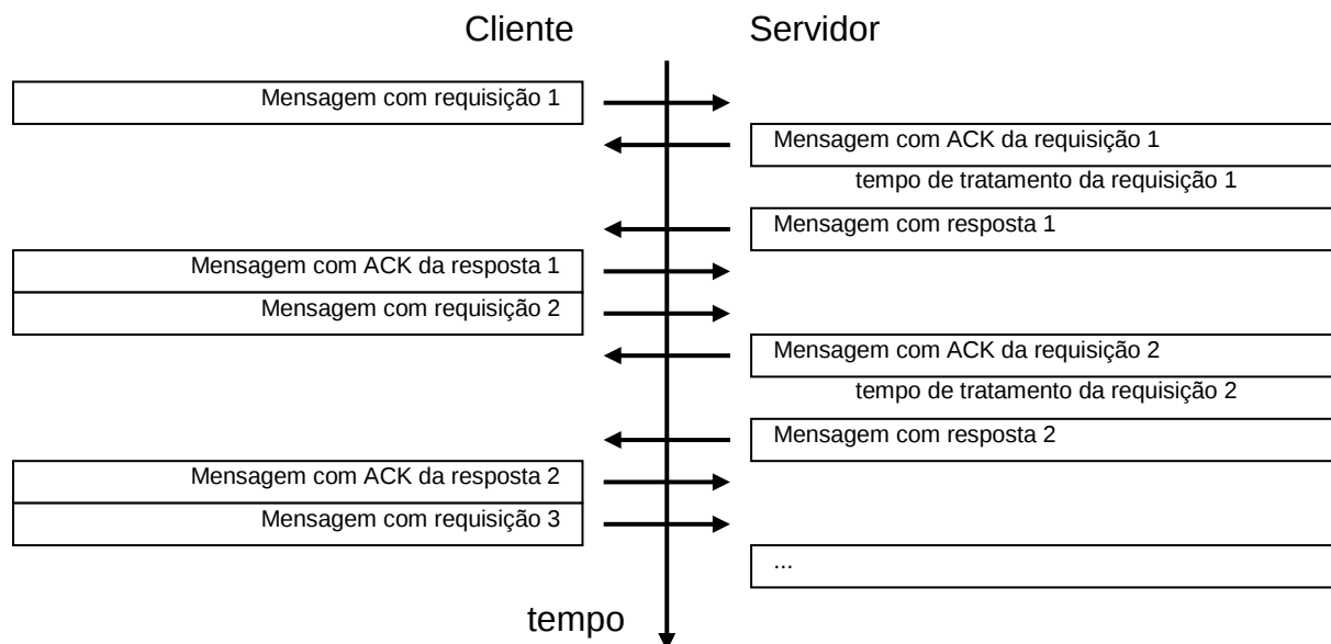
Figura 3-15. Exemplo de funcionamento para envio de ACK imediato (= 0)
