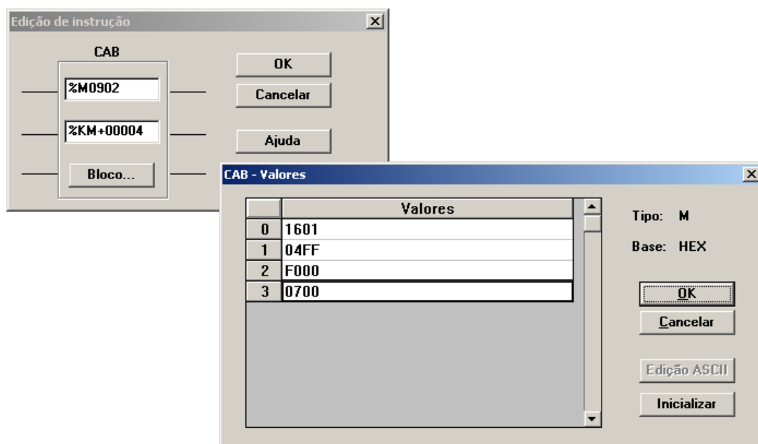
Figura 7-18. Montagem da função nos operandos do CP
