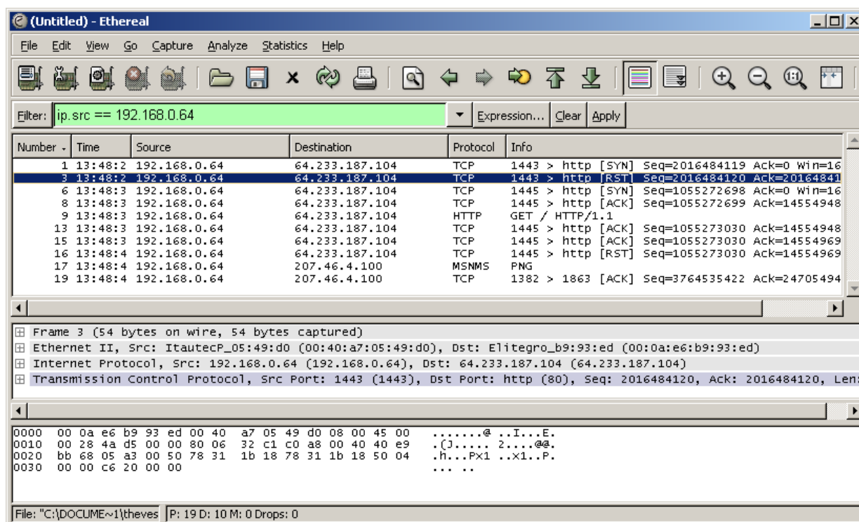
Figura 8-4. Janela de apresentação dos pacotes filtrados
