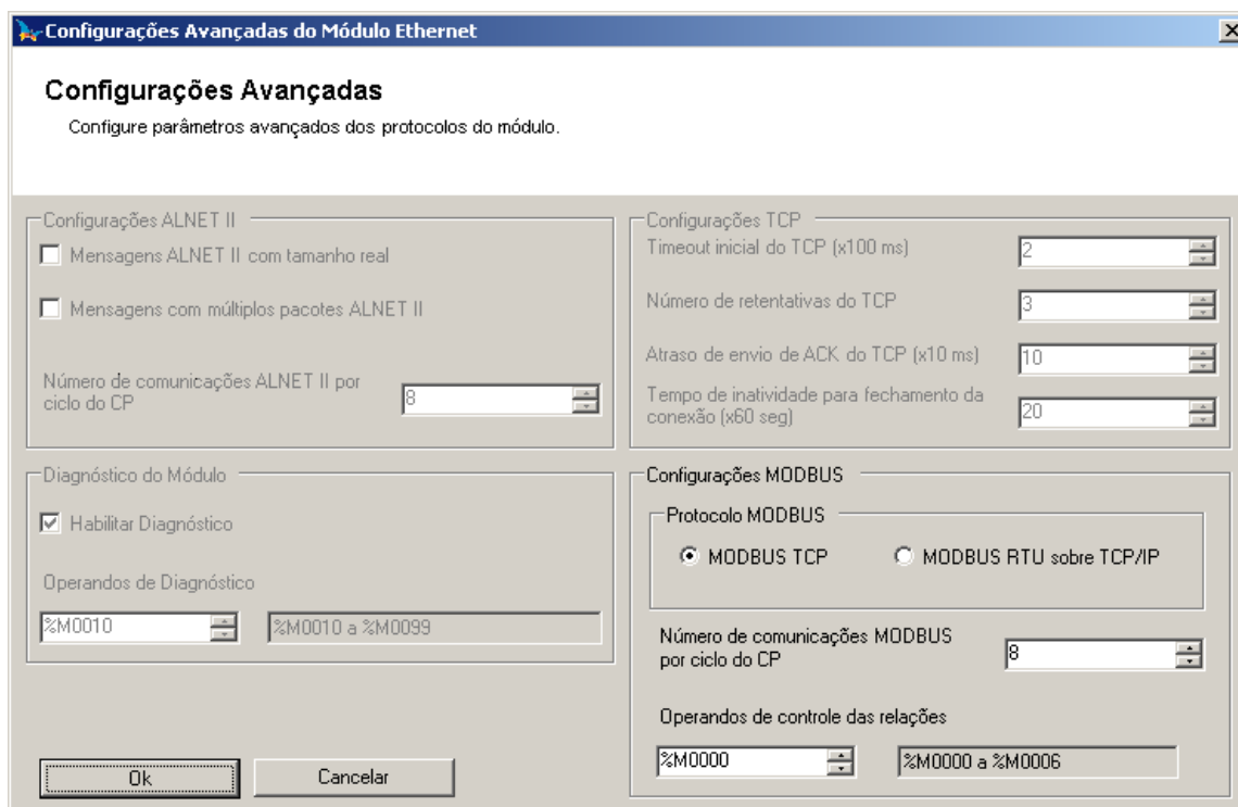
Figura 3-12. Configurações avançadas do protocolo MODBUS
