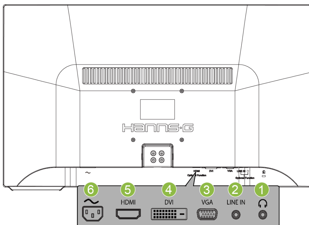
Figura 2. Ligação ao pc
