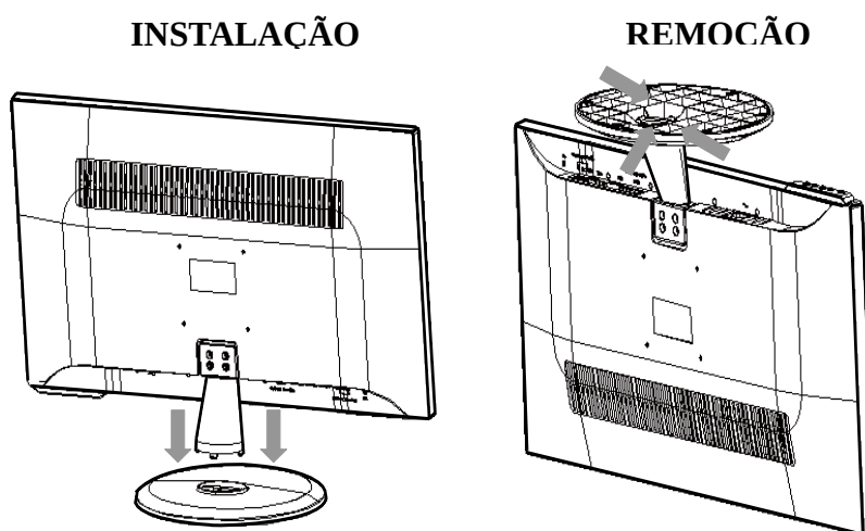
Figura 1. Instalação e remoção da base
