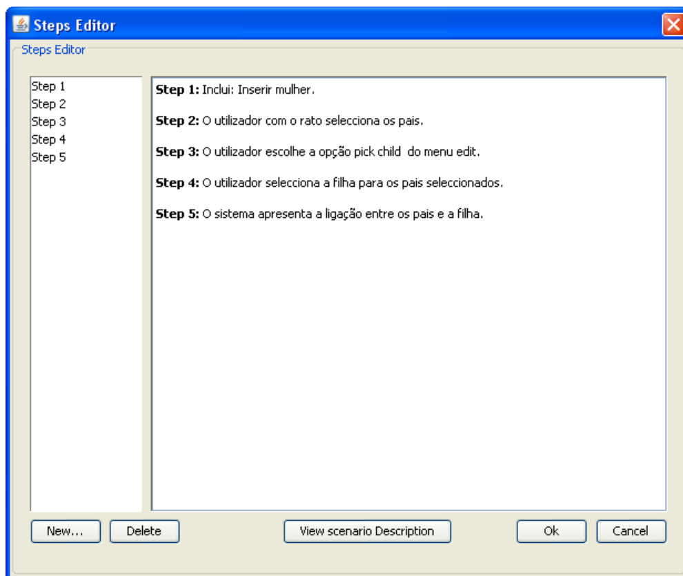
Figura 58 – Edição dos passos do cenário principal do caso de utilização Inserir filha .
