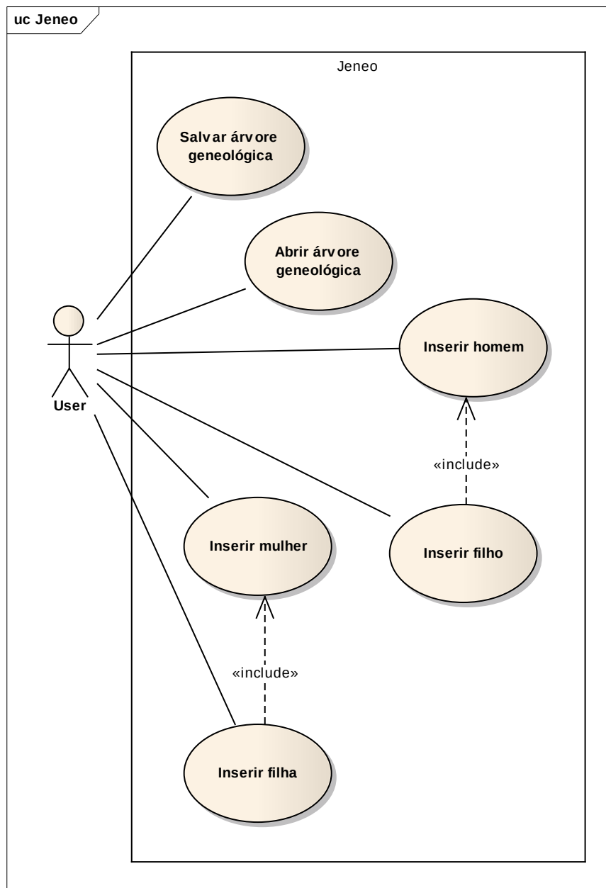
Figura 54 – Casos de utilização do Jeneo
