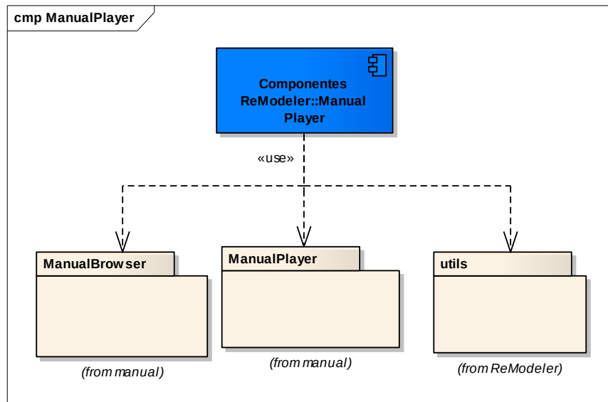
Figura 30 – Pacotes do componente responsável pela visualização do manual de utilizador
