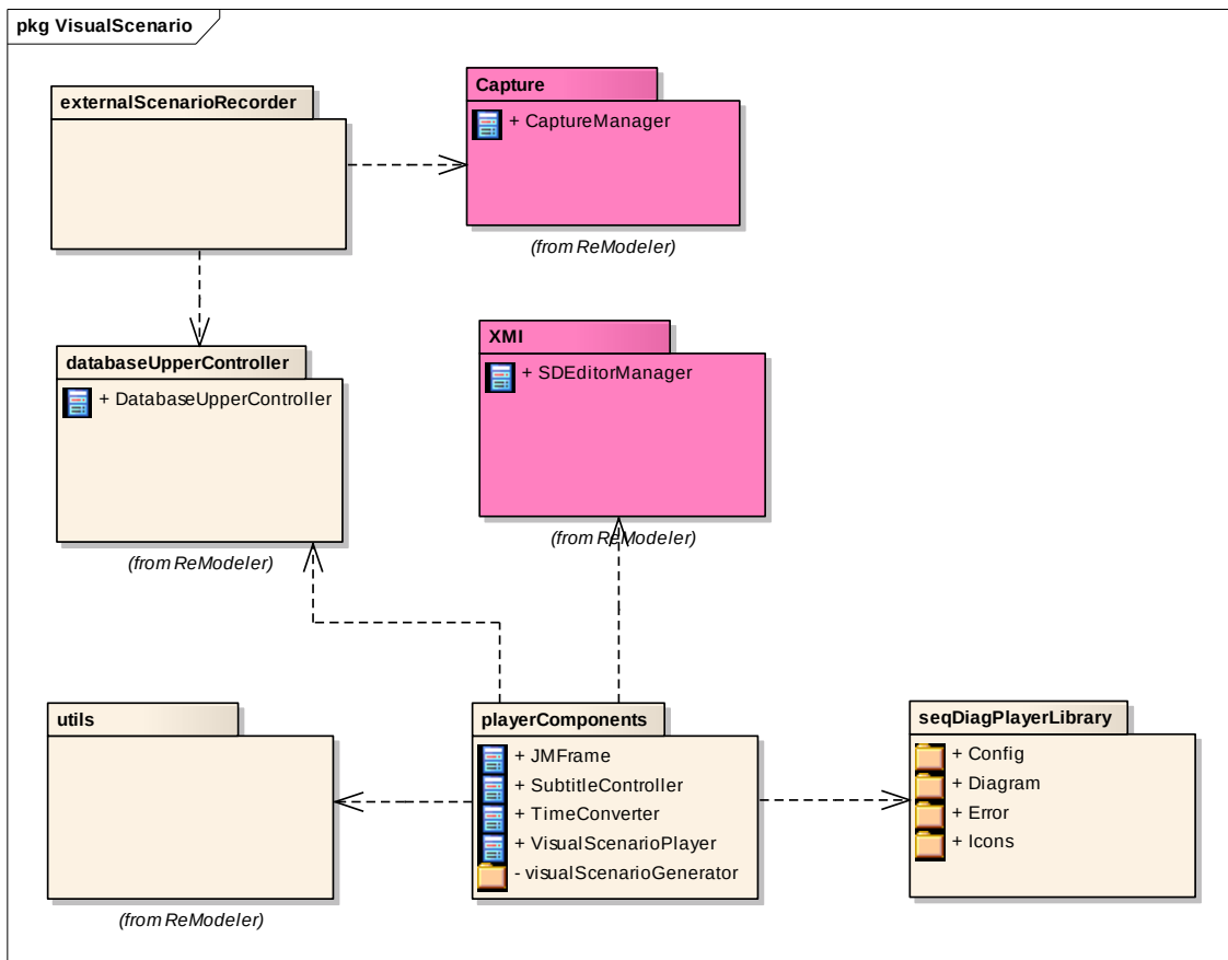
Figura 35 – Diagrama de Pacotes interno do pacote visualScenario .
