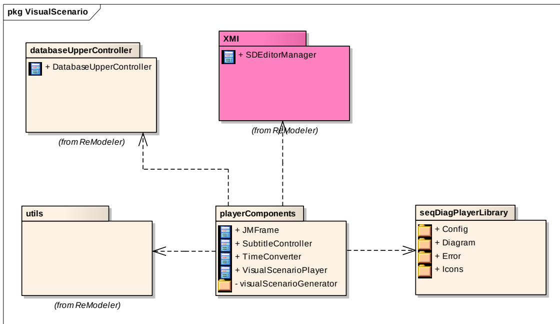
Figura 39 - Pacotes que implementam a geração e reprodução de um cenário visual
