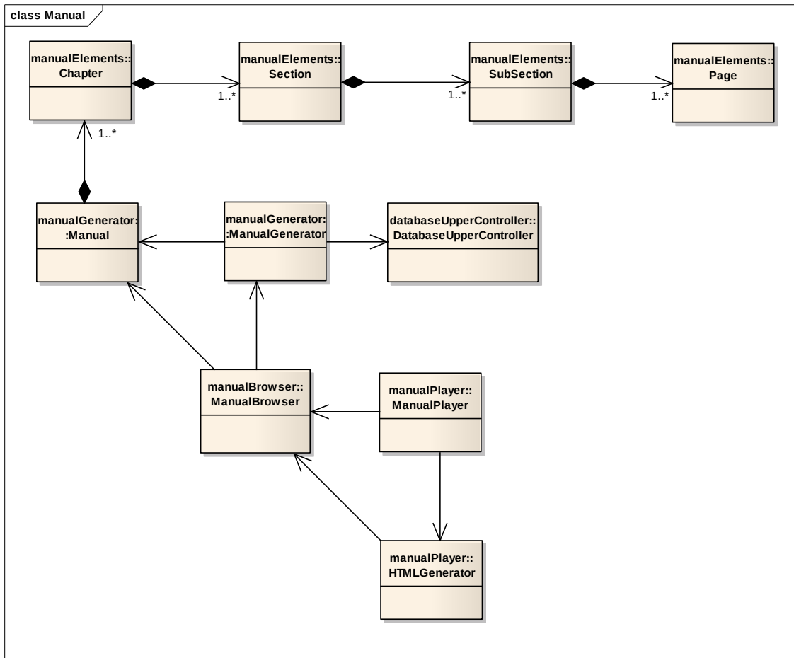
Figura 48 - Diagrama de classes do pacote Manual
