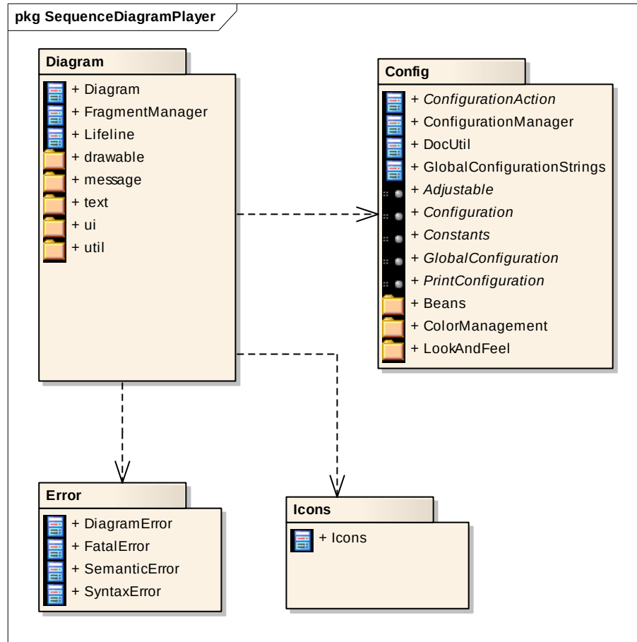
Figura 42 - Diagrama de pacotes da biblioteca de desenho de diagramas de sequência do ReModeler
