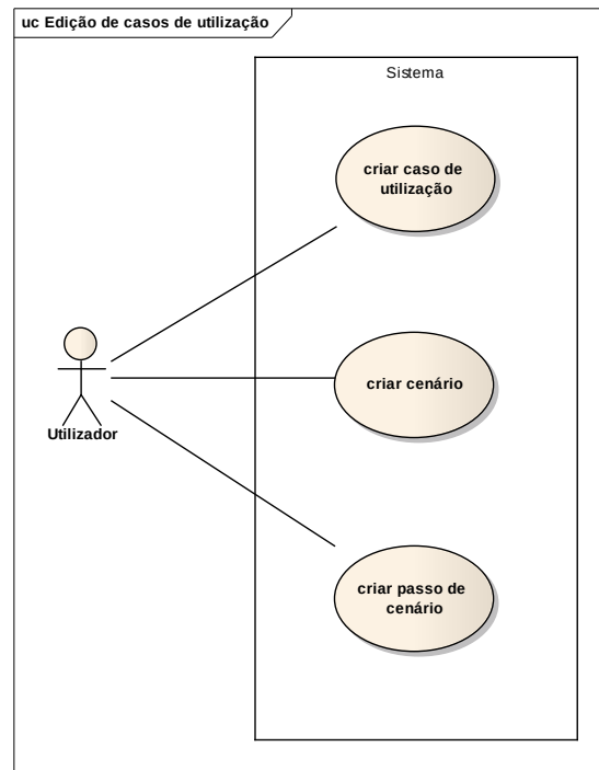
Figura 17 – Casos de utilização para a edição de casos de utilização.
