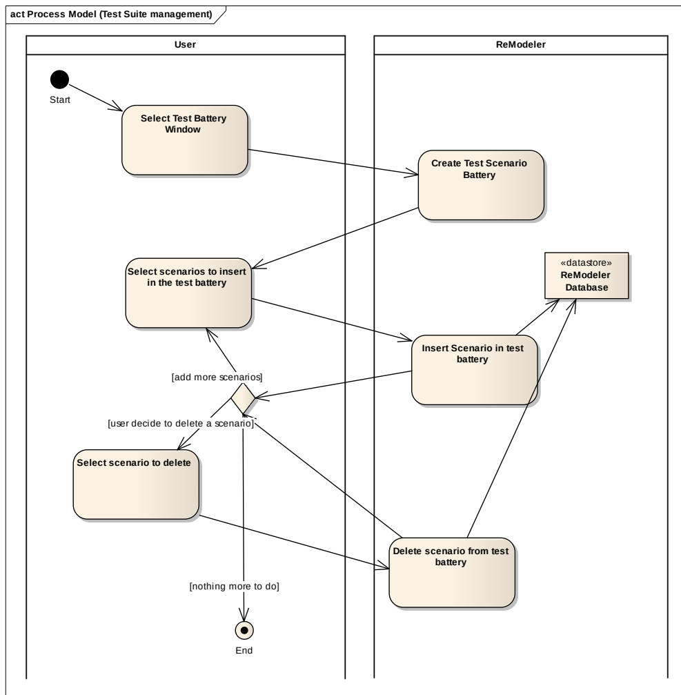
Figura 16 – Diagrama de actividades para a gestão de baterias de cenários de teste
