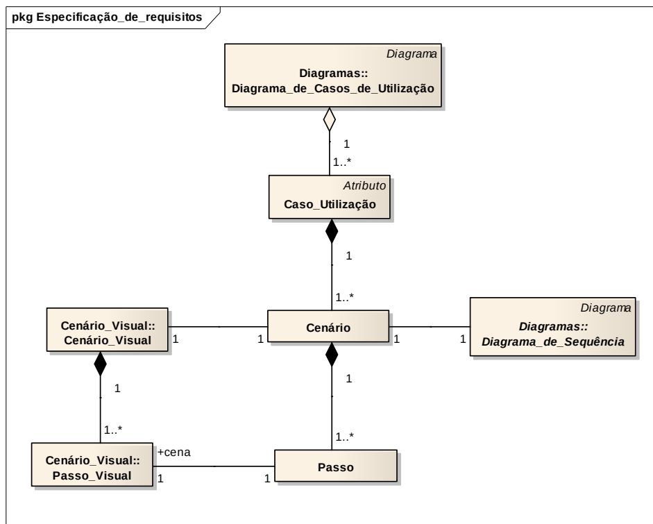
Figura 11 – Fragmento da ontologia do domínio da modelação aumentada (criação de casos de utilização)
