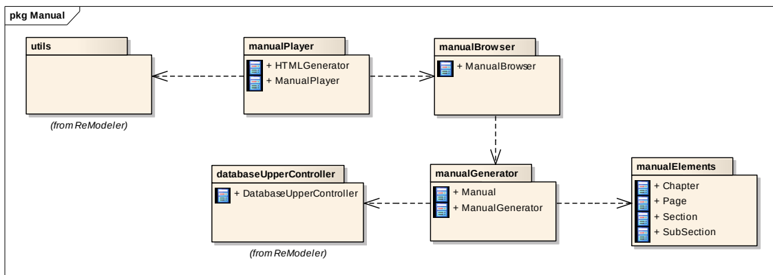
Figura 47 - Diagrama de pacotes do pacote Manual
