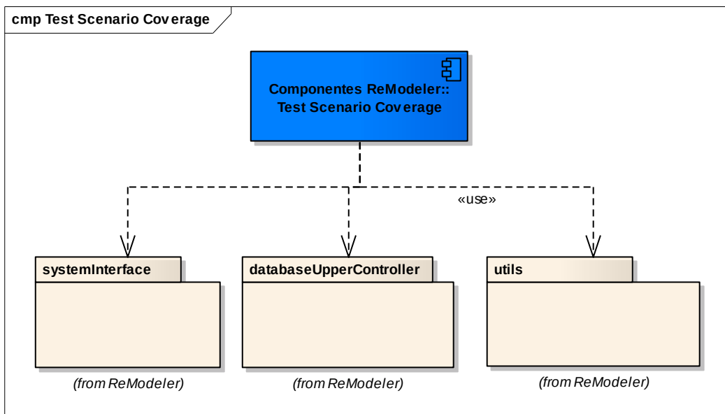
Figura 32 – Pacotes do componente de cobertura de cenários de teste
