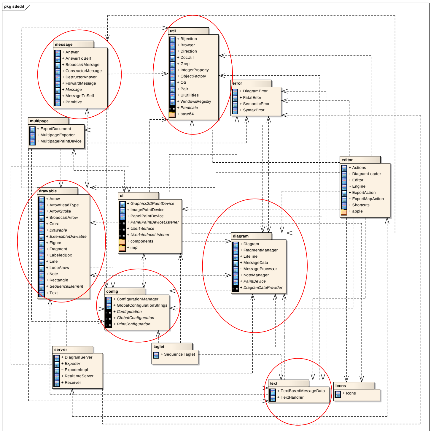
Figura 41 - Diagrama de pacotes do QSDE
