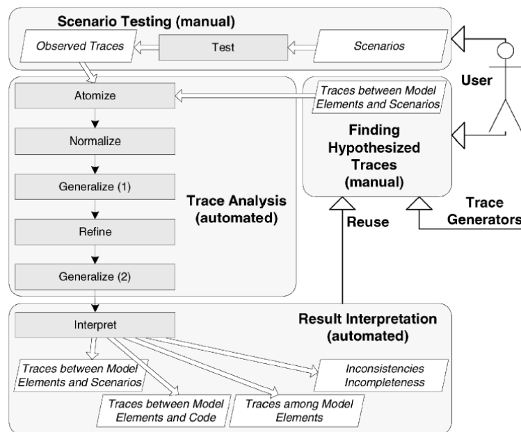
Figura 3 - Visão global das actividades para criação das ligações de rastreabilidade ( em [15] )
