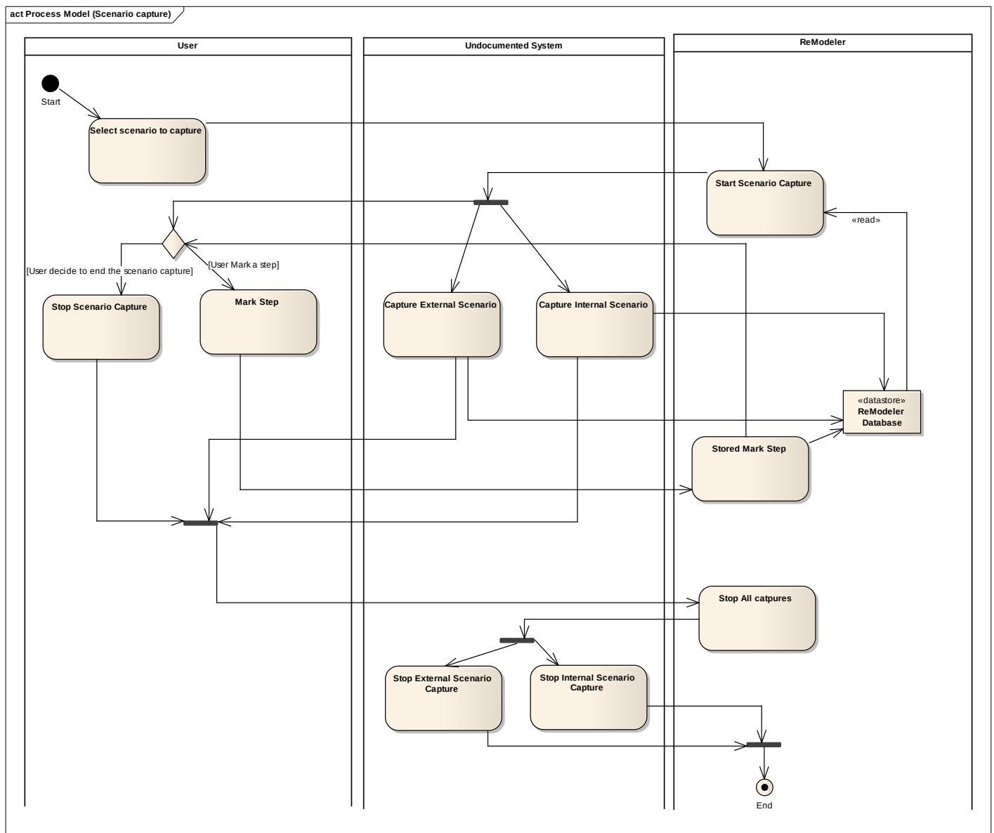
Figura 13 – Processo de captura de cenários
