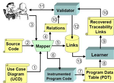
Figura 4 - Arquitectura do LeanArt (em [13] )
