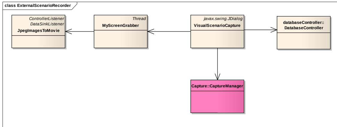
Figura 37 - Diagrama de classes do pacote externalScenarioRecorder
