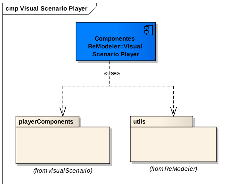
Figura 27 – Pacotes do componente responsável pela reprodução dos cenários visuais
