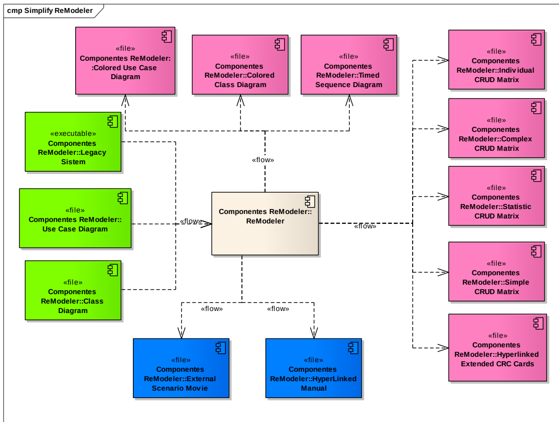
Figura 22 – Os inputs e outputs do ReModeler .
