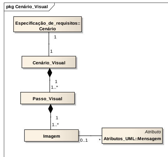
Figura 7 - Fragmento da ontologia do domínio da modelação aumentada (cenário visual)
