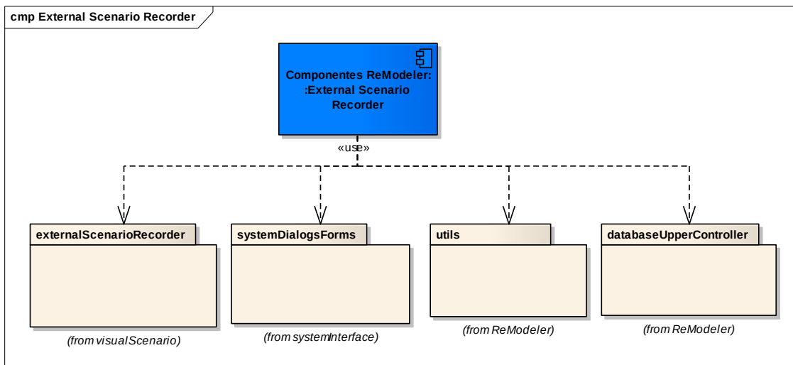
Figura 25 – Pacotes do componente de captura de cenários externos.
