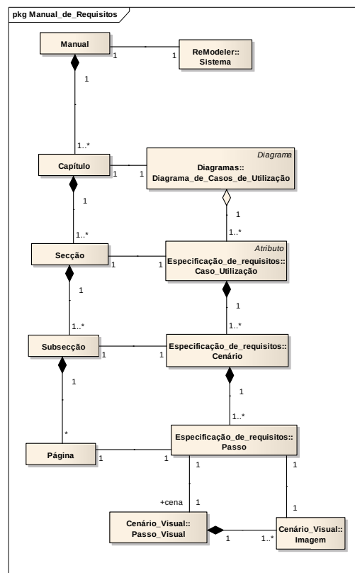
Figura 8 – Fragmento da ontologia da modelação aumentada (manual de utilizador)
