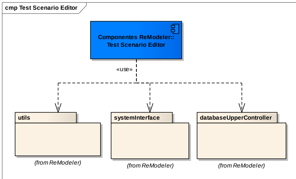
Figura 31 – Pacotes do componente de edição de cenário de teste
