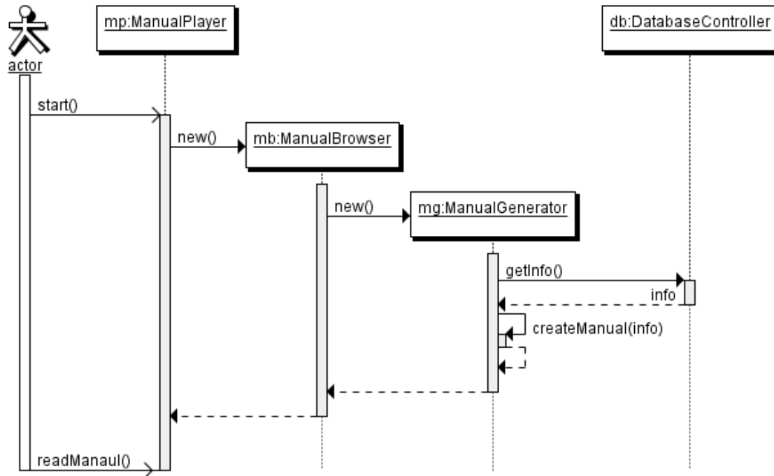
Figura 49 - Diagrama de sequência da geração e visualização do manual de utilizador
