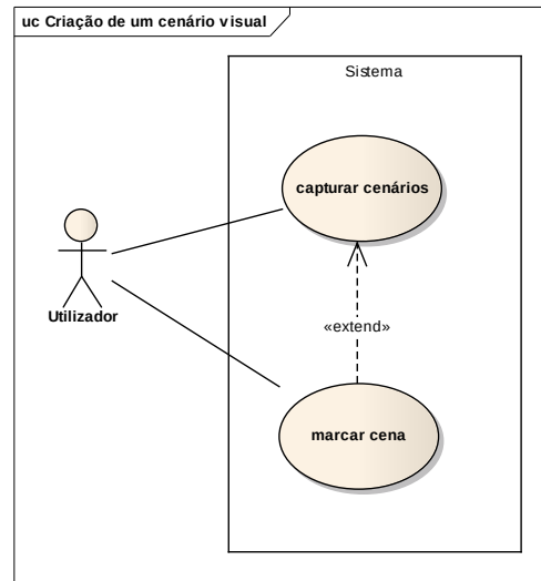
Figura 18 – Casos de utilização para a captura de cenários.
