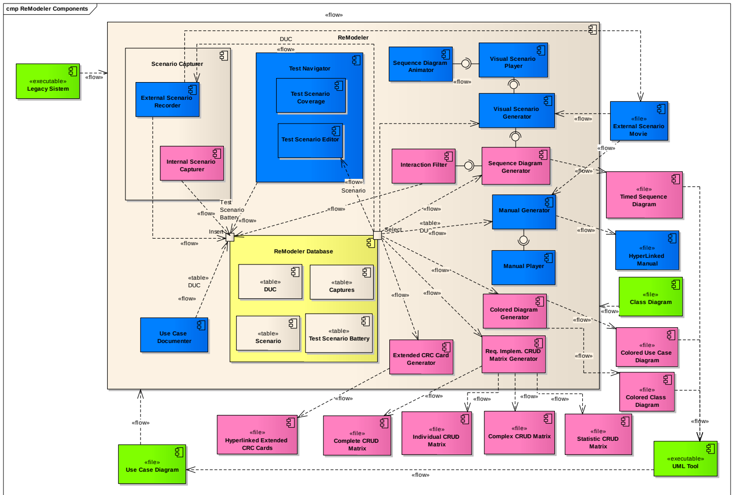
Figura 23 – Diagrama de componente do ReModeler
