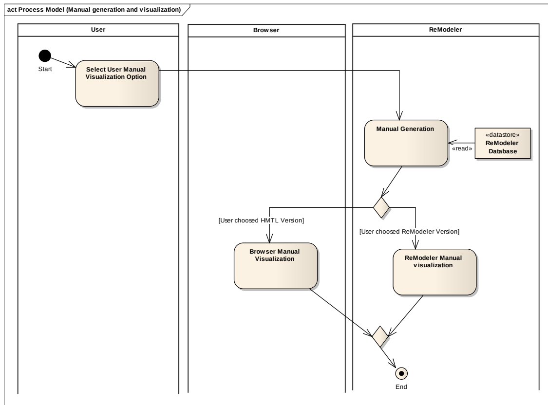
Figura 15 – Diagrama de actividades para a geração e visualização do manual.
