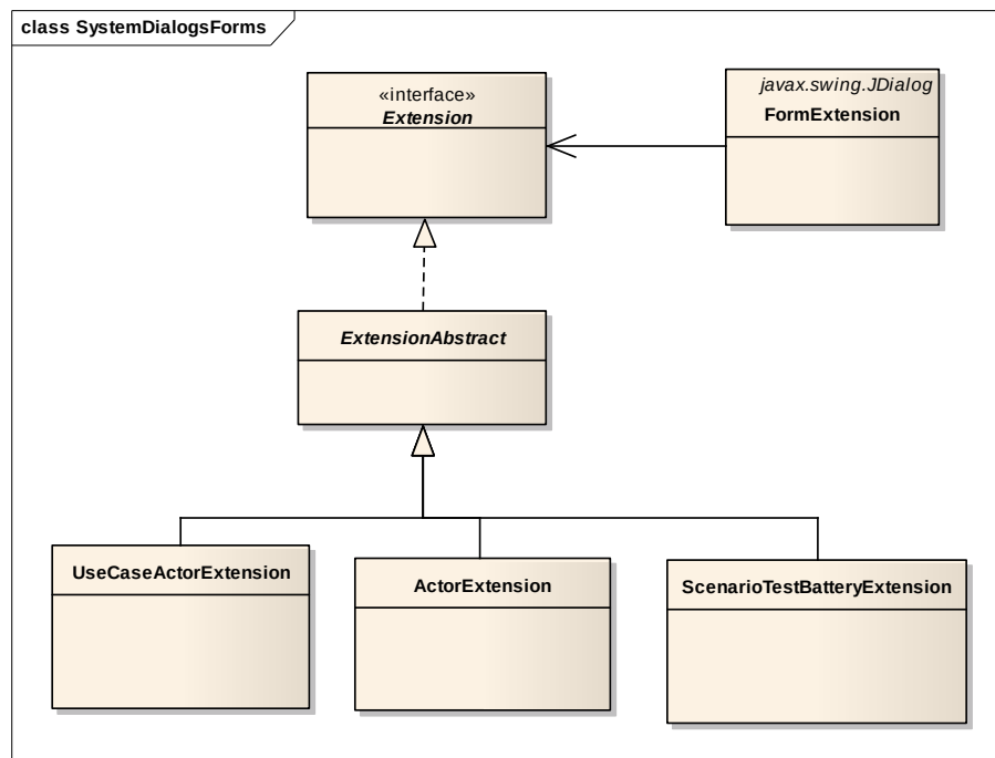
Figura 52 - Excerto do diagrama de classes do pacote systemDialogForms
