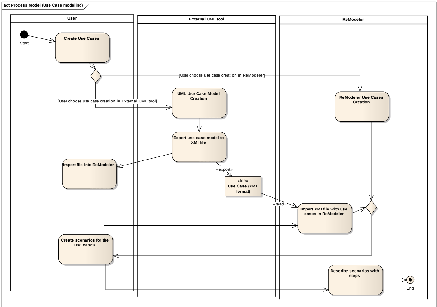
Figura 12 – Criação de casos de utilização
