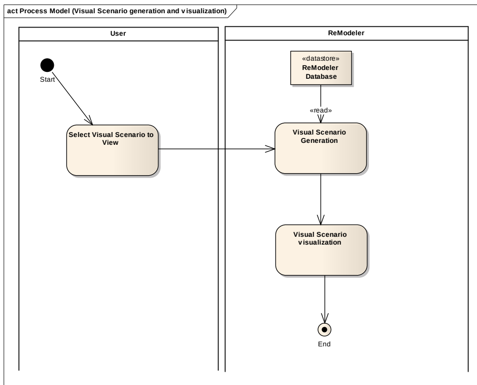
Figura 14 – Diagrama de actividades da criação e visualização de um cenário visual
