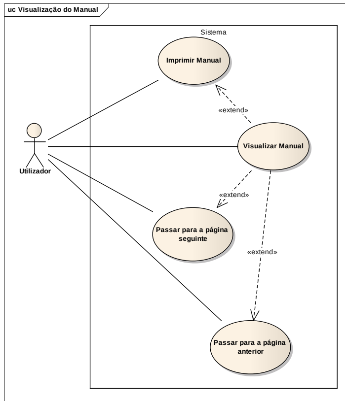
Figura 20 – Casos de utilização para o manual de utilizador.
