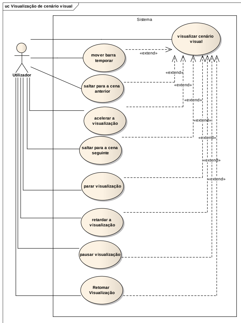
Figura 19 – Casos de utilização para a visualização de cenários visuais.
