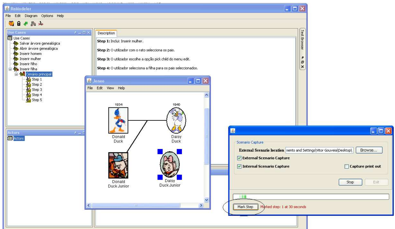
Figura 62 - Marcação de passos do cenário principal do caso de utilização Inserir filha .
