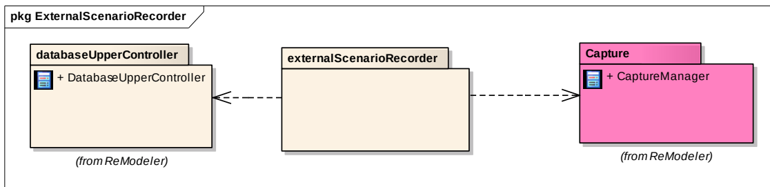
Figura 36 – Diagrama de pacotes relativo à captura de cenários.
