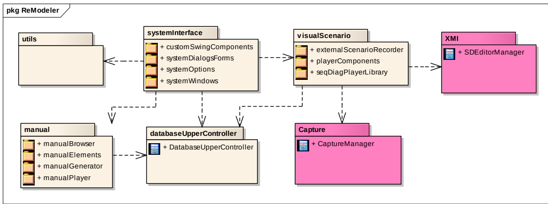
Figura 33 – Diagrama de pacotes global
