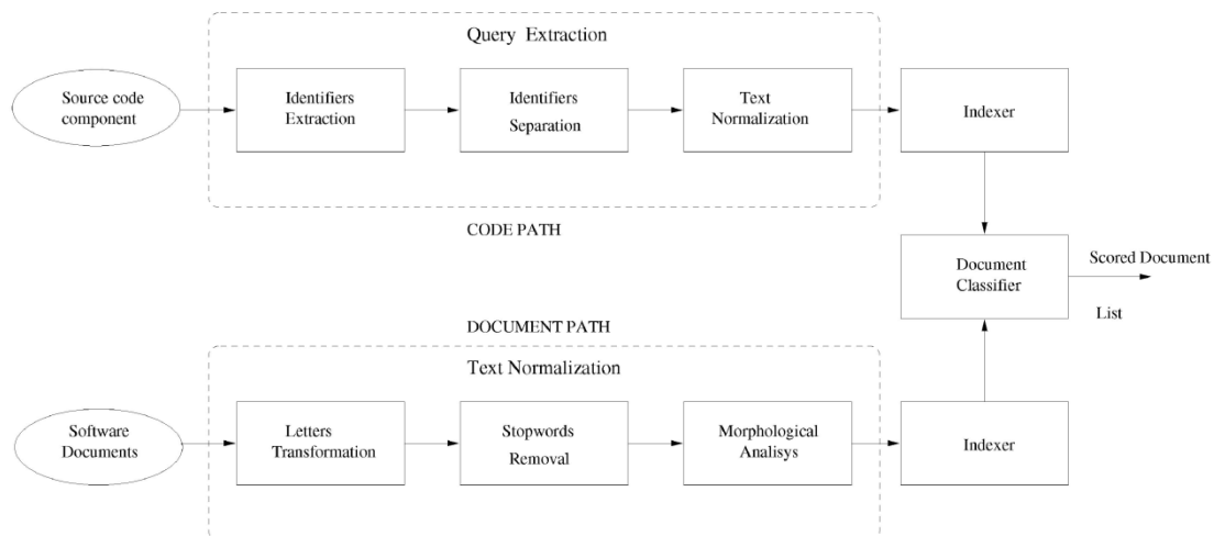
Figura 1 - Método de geração das ligações de rastreabilidade (em [21] )
