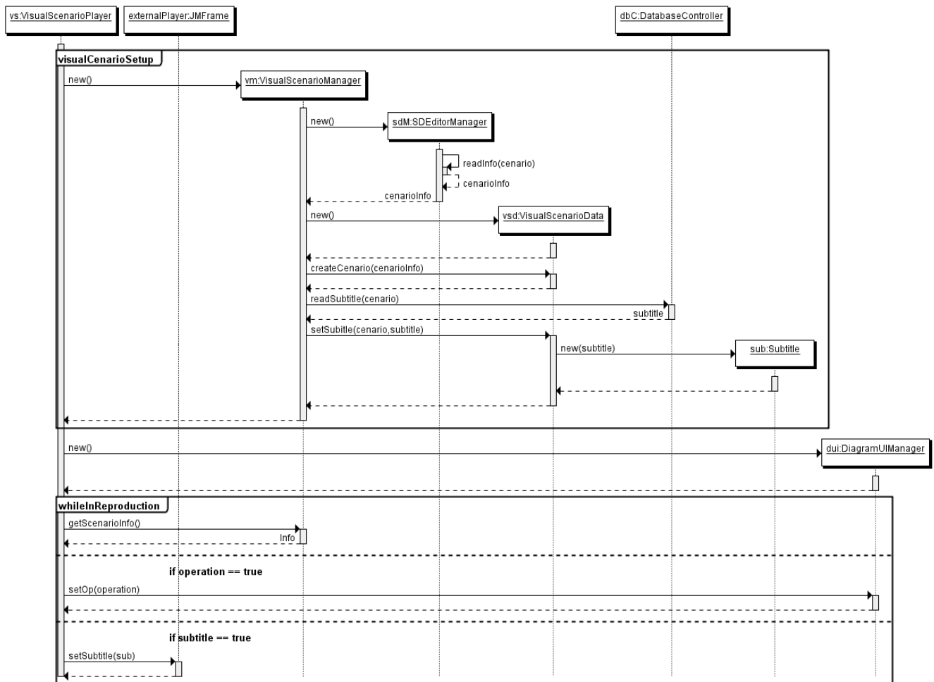
Figura 46 - Diagrama de sequência da geração e reprodução de um cenário visual
