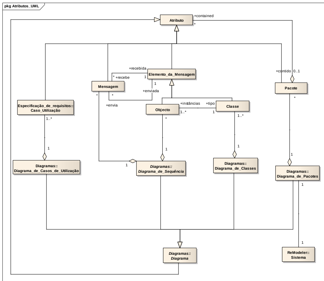
Figura 9 – Fragmento da ontologia do domínio da modelação aumentada (conceitos UML)
