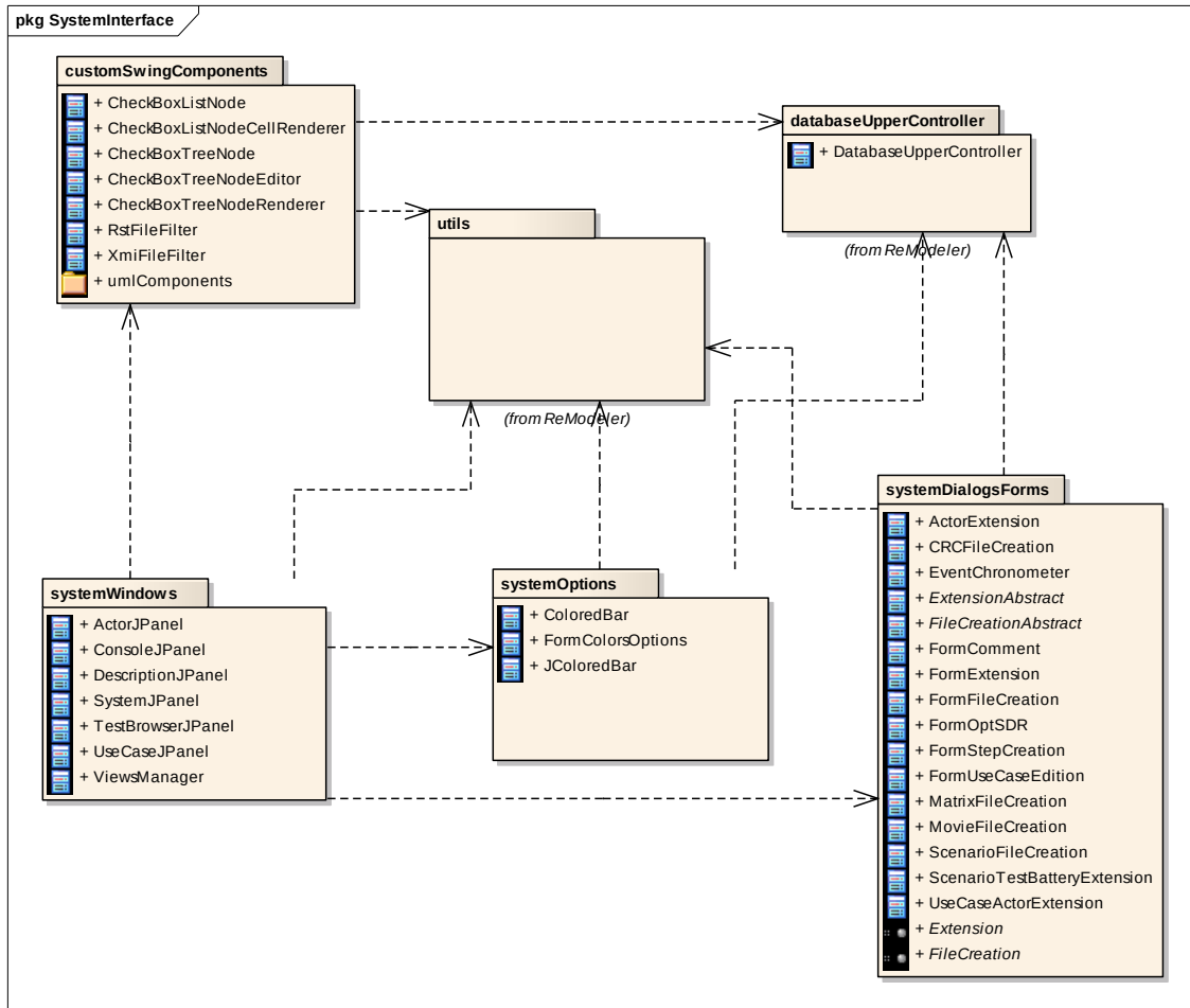
Figura 50 - Diagrama de pacotes do pacote systemInterface
