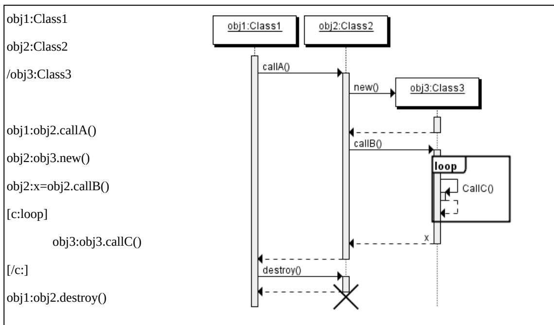
Figura 43 - Diagrama de sequência sem marcação de passos
