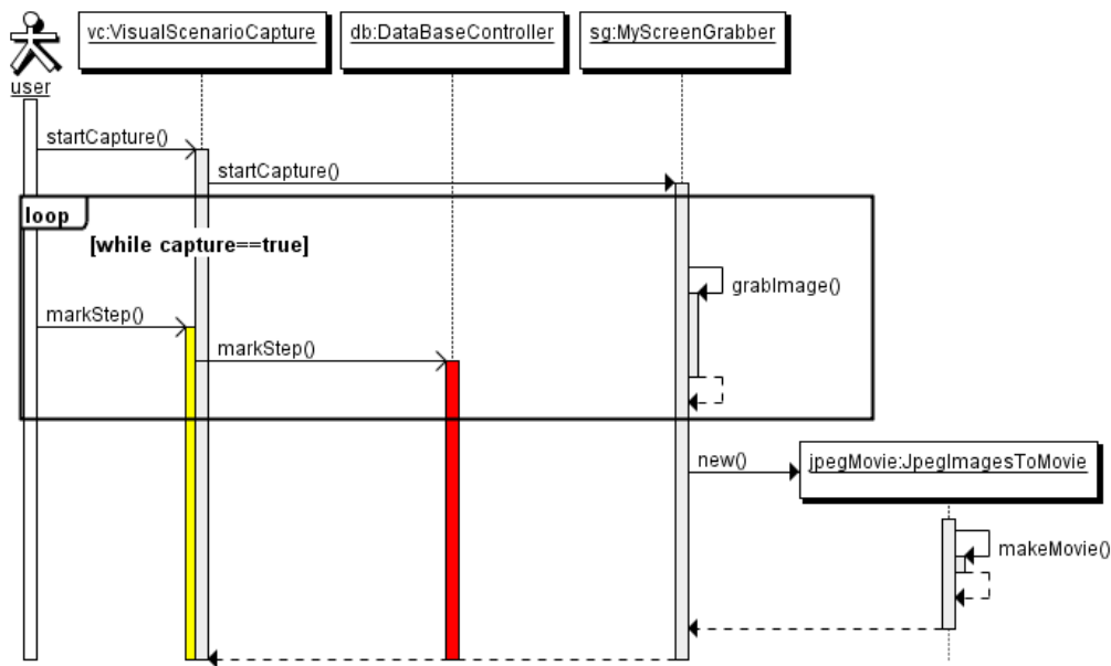
Figura 38 - Diagrama de sequência para captura de um cenário externo
