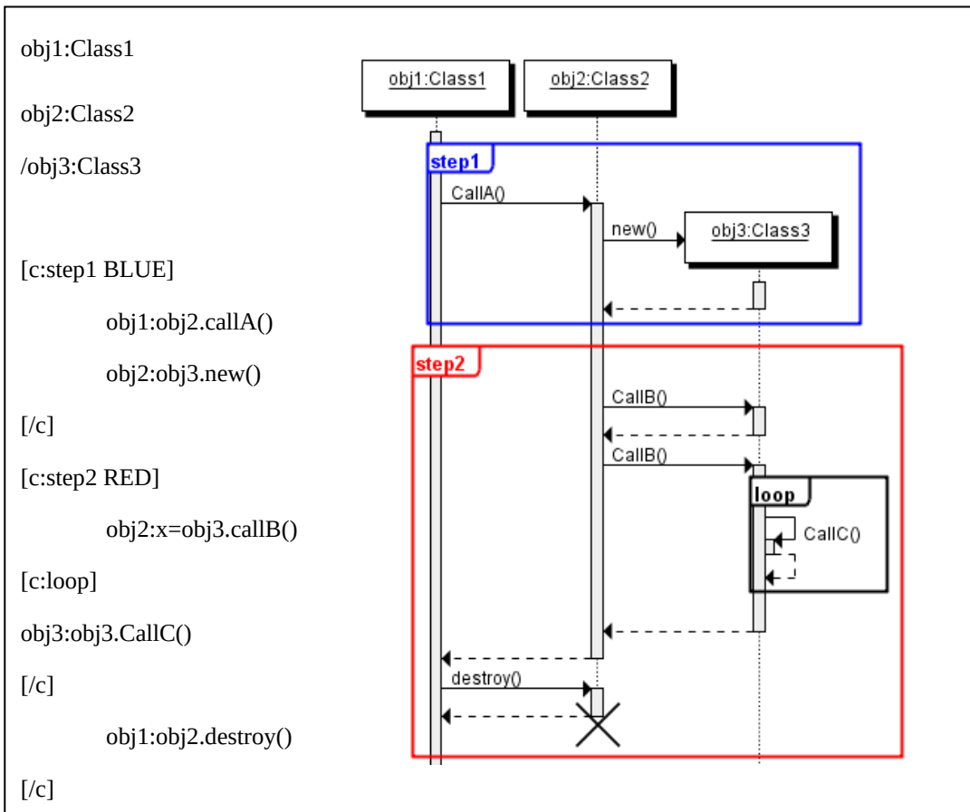
Figura 44 - Diagrama de sequência com marcação de passos de cenário
