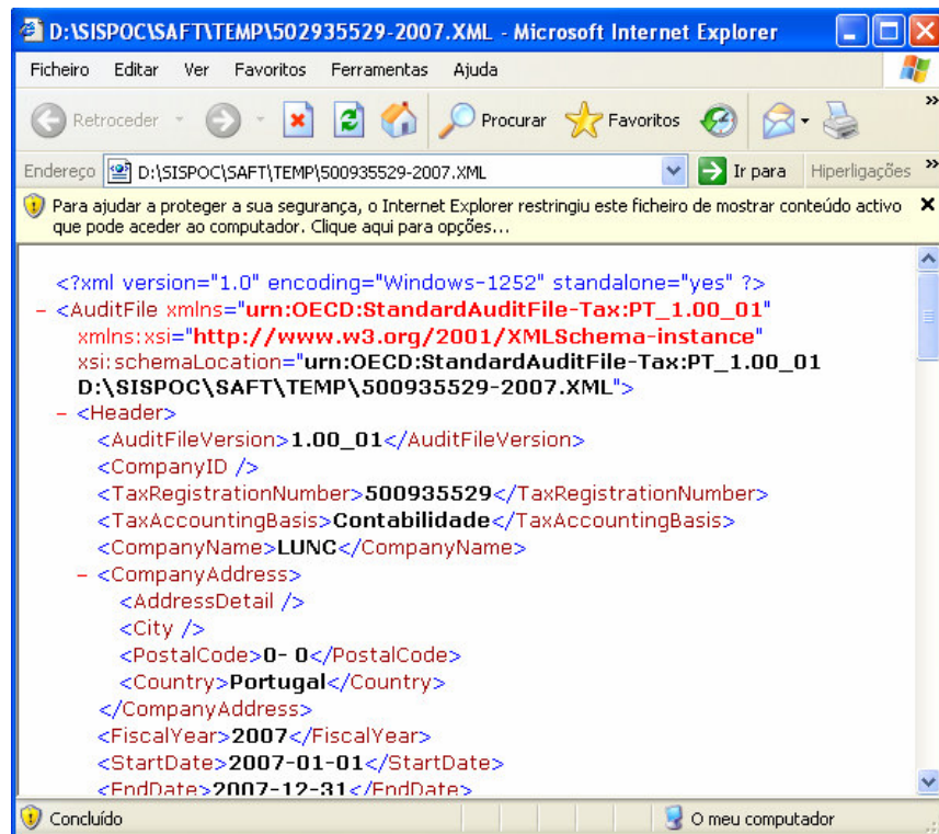
Figura 21 Amostra de ficheiro SAFT
