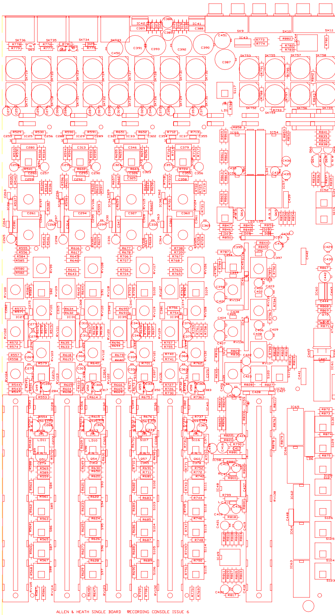
PCB fig.II
