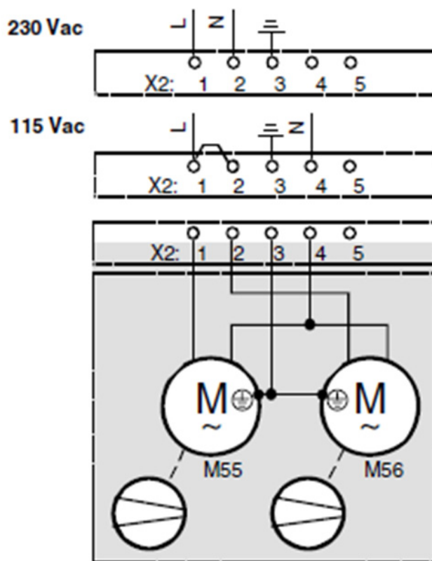
Fan configuration D1 to D3
