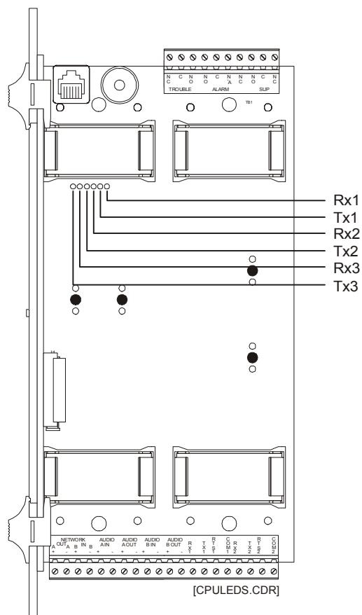
Figure 8-1: CPU module
