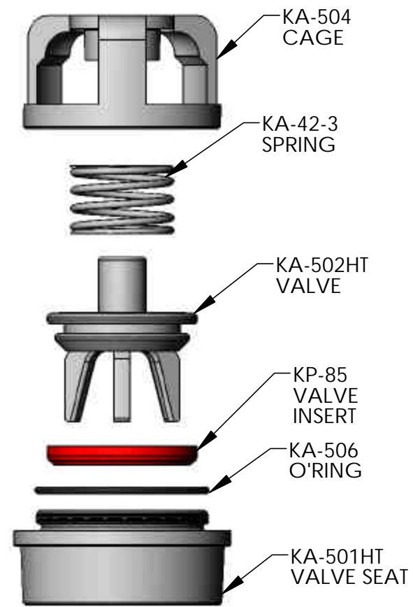
OPTIONAL KA-500HT VALVE ASSEMBLY
