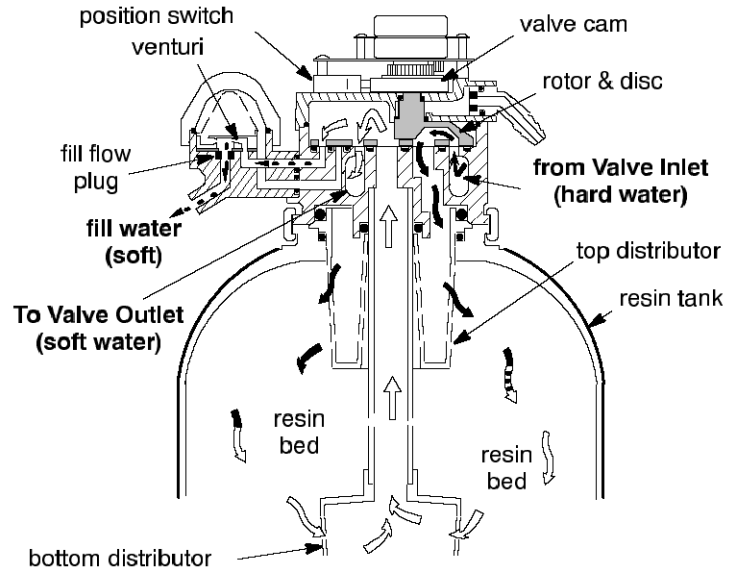
FILL CYCLE
