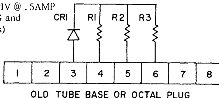
Fig. 13 Calibration Module
