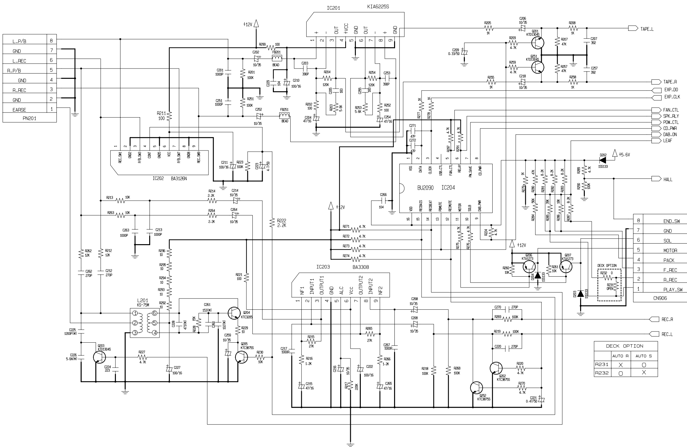
D- SCHEMATIC DECK 3854R11102A (6870R3955AA) LX-W550 LX-(B)W250 3/4
