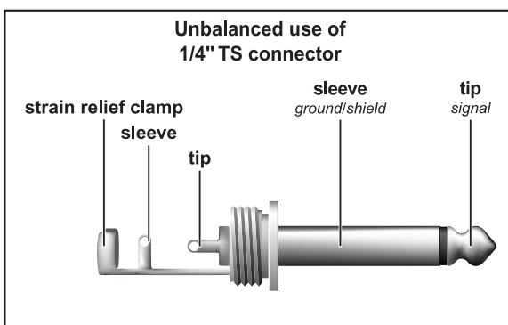
Fig. 4.2: 1/4" mono jack
