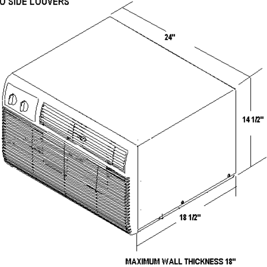
18.5" --NO SIDE LOUVERS
