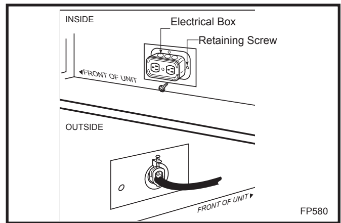
Fig. 6 EB-1 receptacle.
