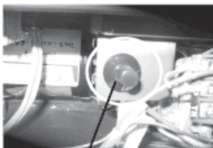
Piezo Ignitor
