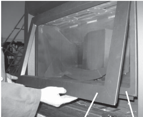
Door Frame Glass Door
