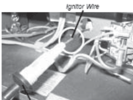
Piezo Ignitor
