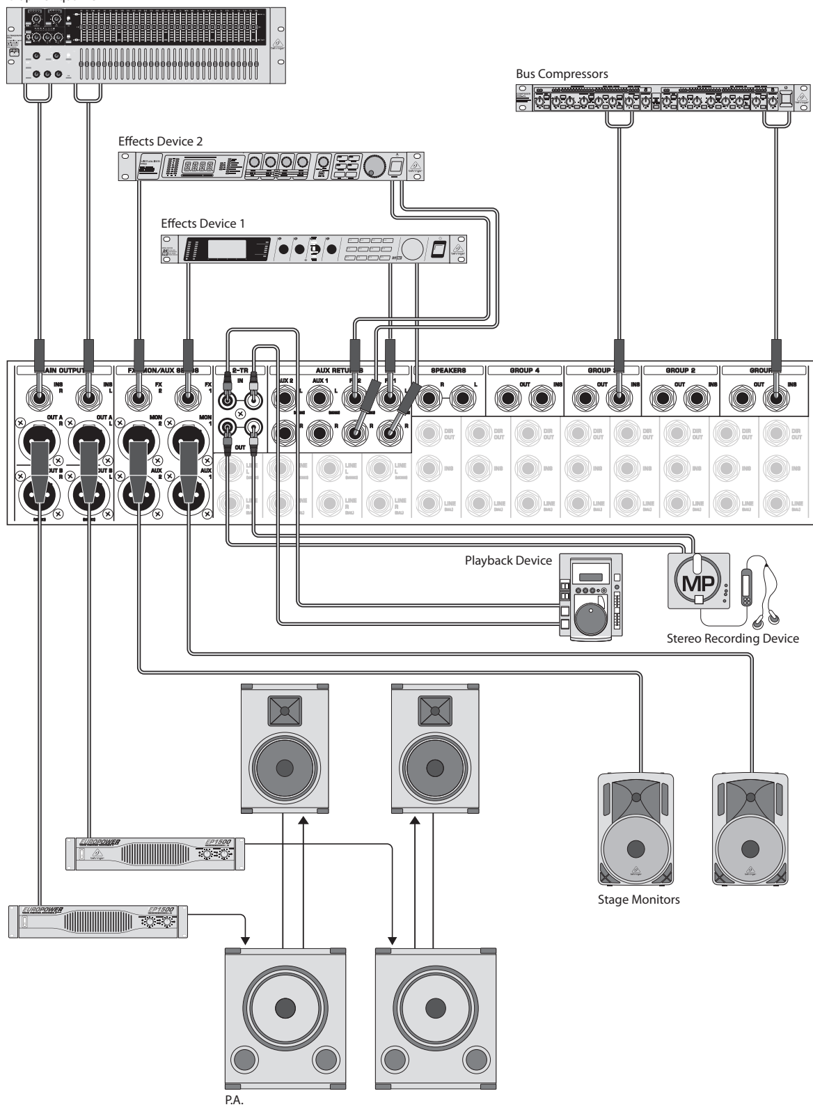
Fig. 2.2: Output wiring
