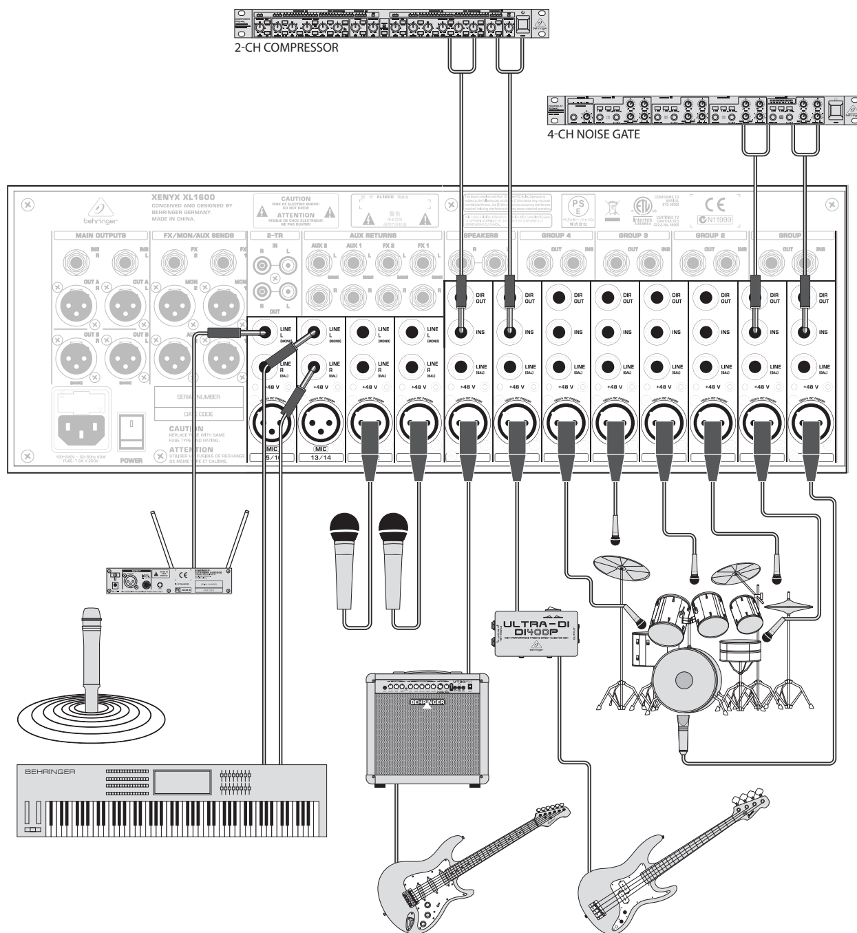
Fig. 2.1: Input wiring
