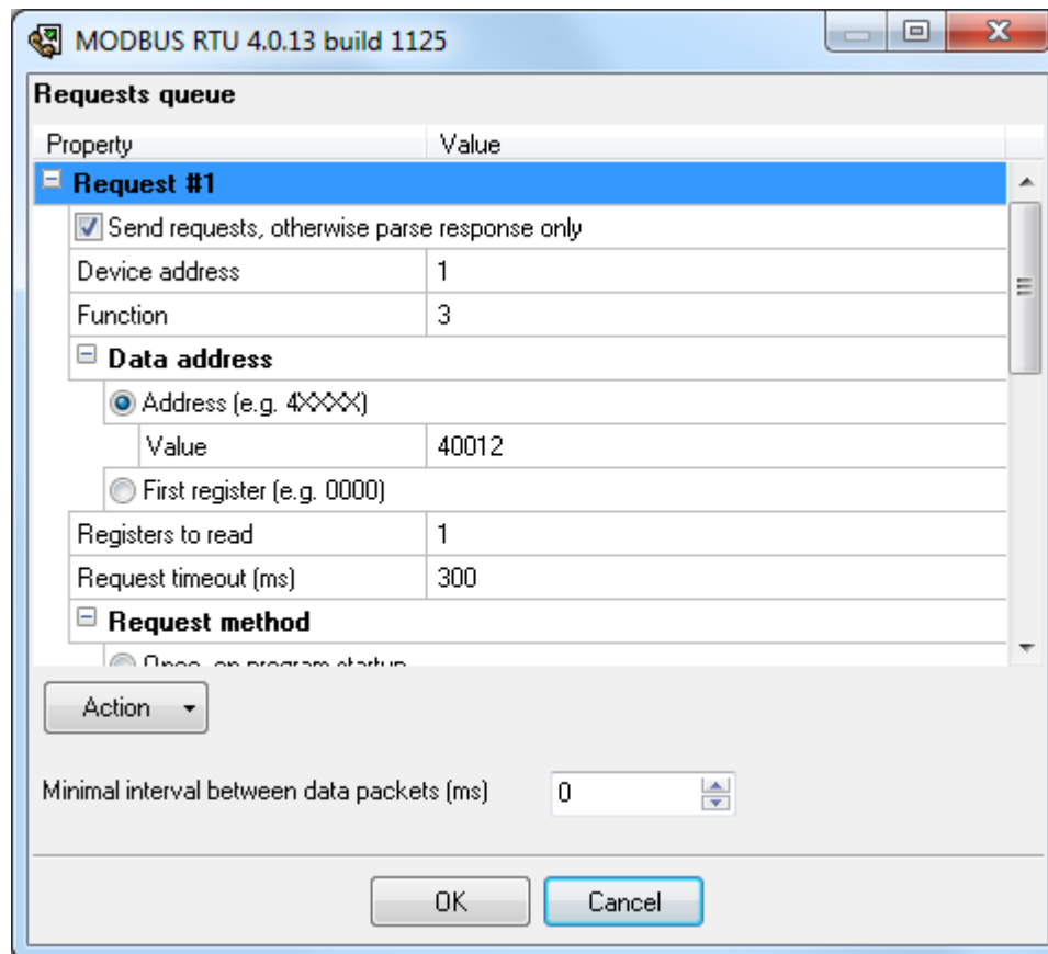
Fig.2. MODBUS request
