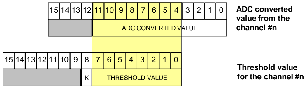
Fig. 5.3: Zero suppression
