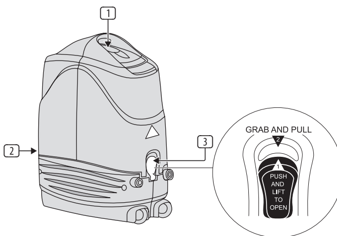
Fig. 2.1: EPA900 setup
