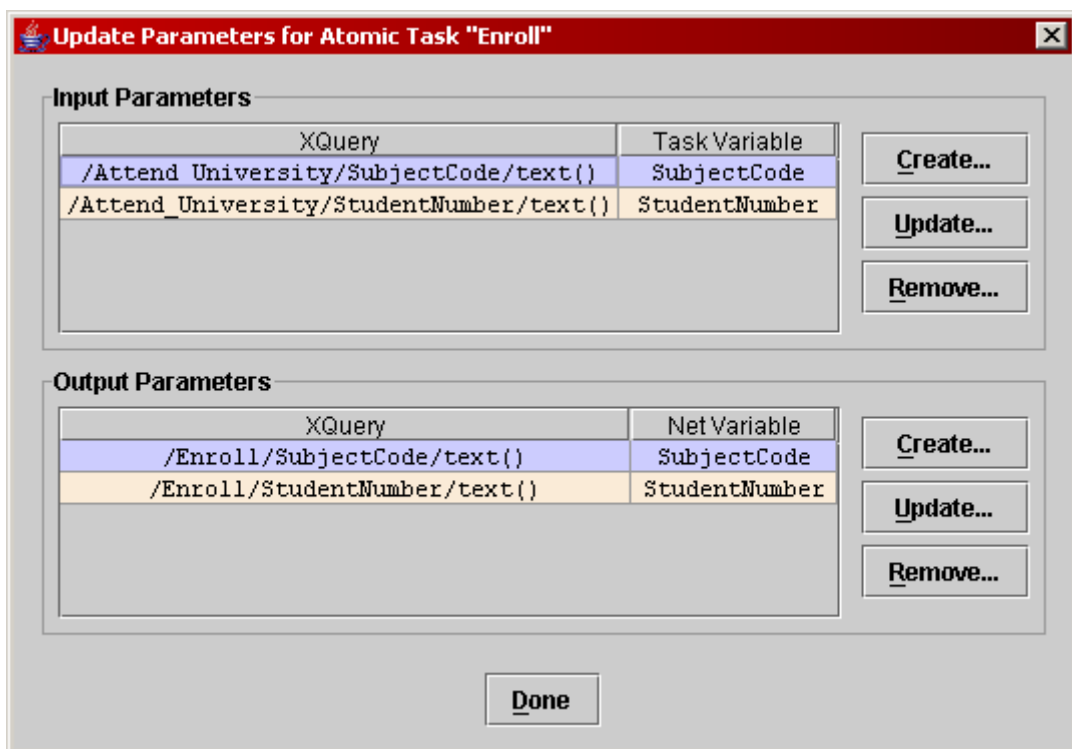
Fig. 31. Established task parameters
