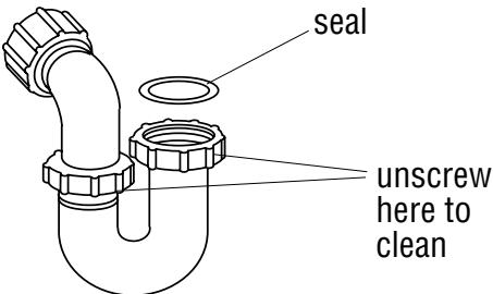
U-bend trap
