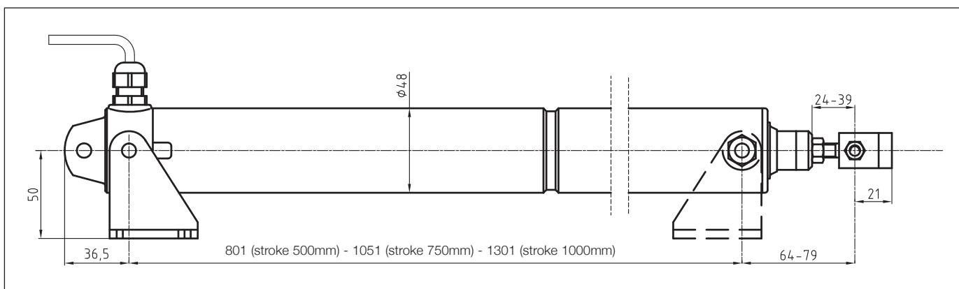
Actuator dimensions
