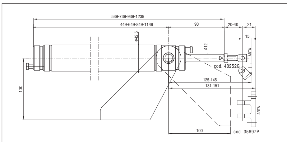
Actuators dimensions
