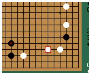
Figure 12.10.: Goban
