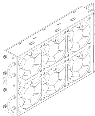
Figure 3-21 Fan Tray 4U
