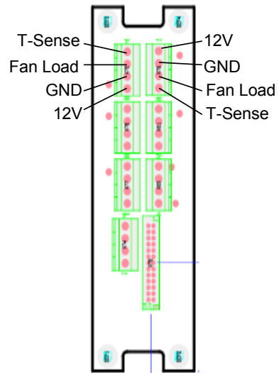
PCB Fan Tray Interface
