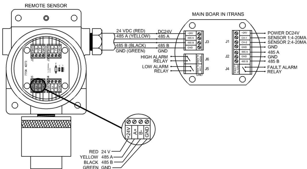
Figure 4-7. Wiring Remote Sensors Back to iTrans™ ERREUR ! SOURCE DU RENVOI INTROUVABLE.
