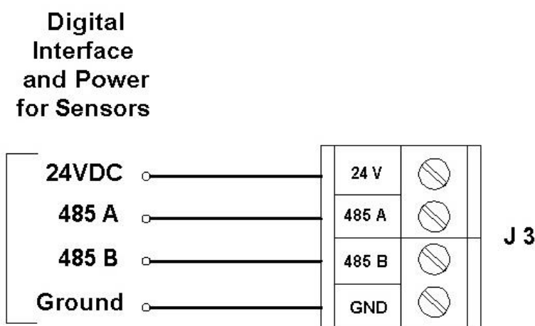
Figure 4-3. Sensor Connector J3 on the iTrans ™ ERREUR ! SOURCE DU RENVOI INTROUVABLE .
