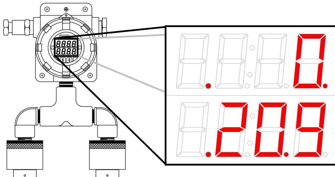
Figure 2-2. The iTrans™ ERREUR ! SOURCE DU RENVOI INTROUVABLE . Display (Dual-Gas Monitor Shown)
