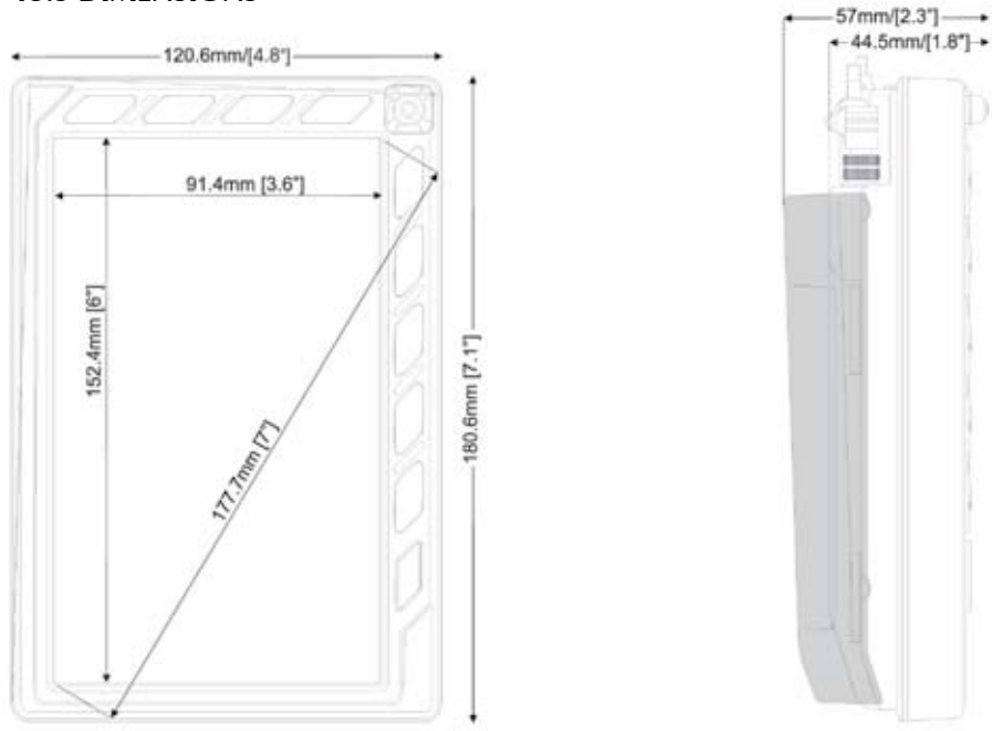
Fig. 15.3 - Dimensions
