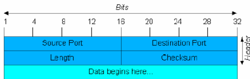
UDP Datagram
