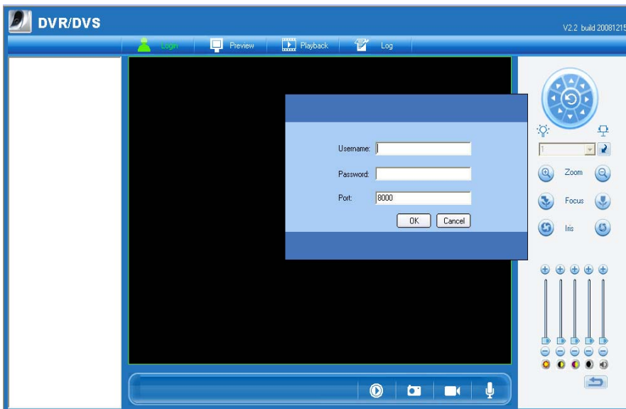
Fig. 3.4 Login Interface
