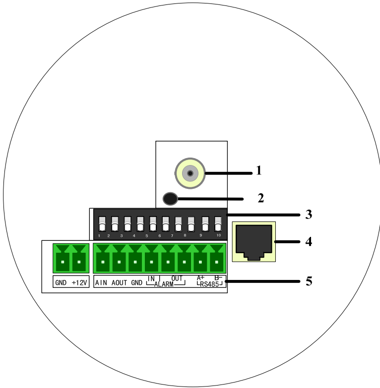
Fig. 2.1.6 Rear Panel of DS-2CD752 、 DS-2CD762 series
