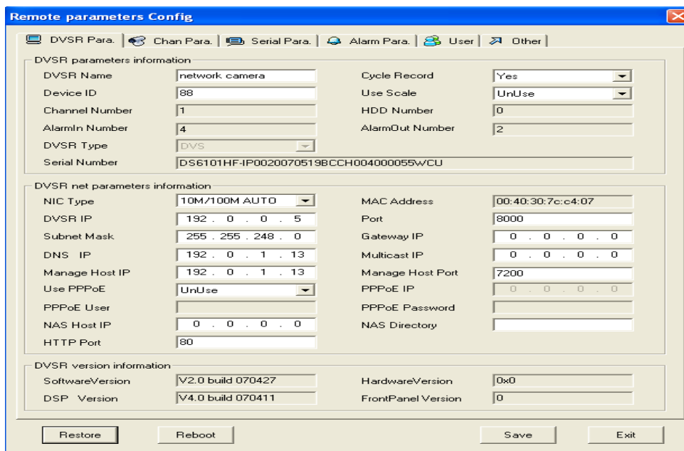
Fig. 3.6 Remote Parameters Configuration
